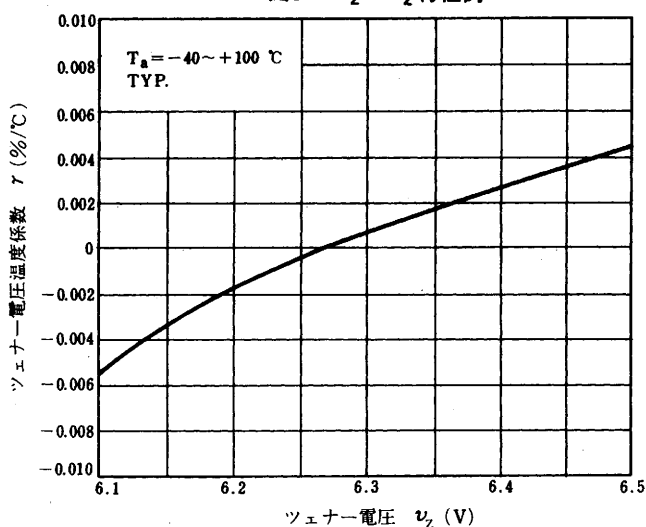
図2. r_z - v_z 特性例
