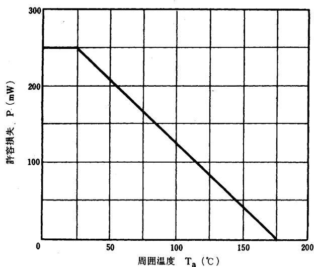
図1. P-T_a 定格
