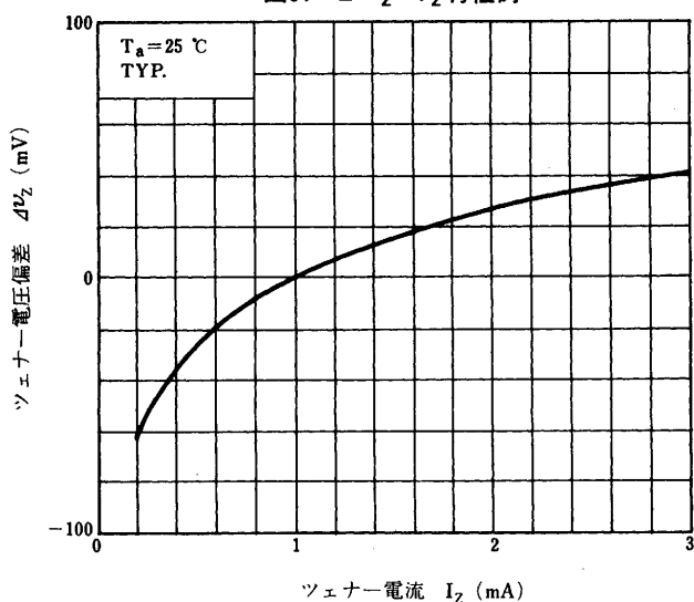
図3. \Delta v_z - i_z 特性例
