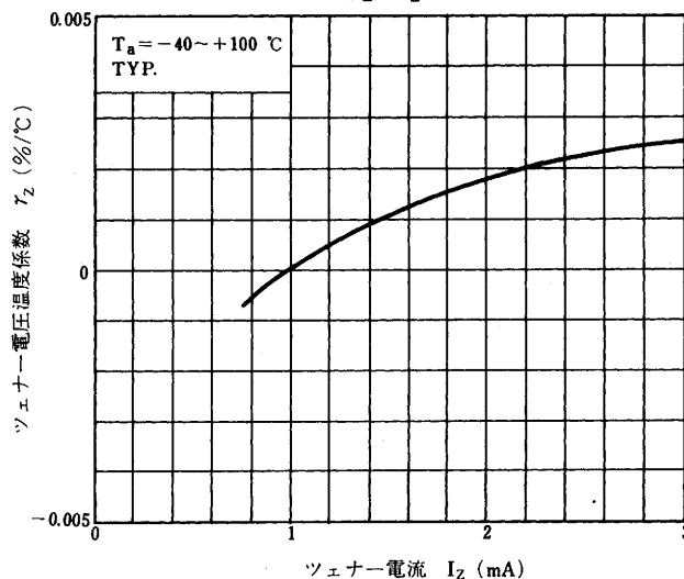
図4. r_z - i_z 特性例
