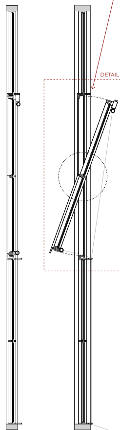
Detail 3 Scale: 3"=1'
