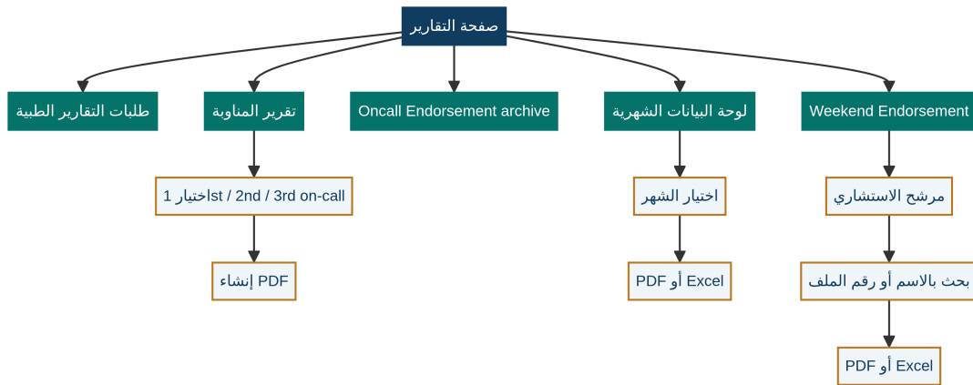
图 6 مسار تقرير Weekend Endorsement: اختيار الاستشاري، البحث، ثم تصدير PDF أو Excel.
