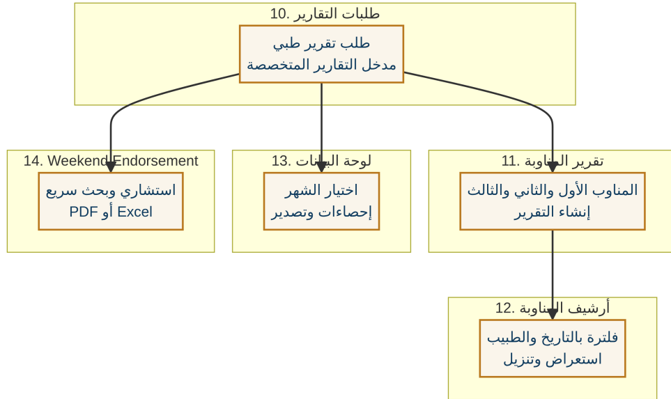
5 图 خريطة صفحات التقارير: طلبات التقارير والمناوبة والأرشفة ولوحة البيانات وWeekend Endorsement.
