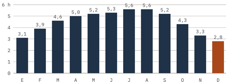
Figura 2.1. Horas de sol pico al día por mes a 42^\circ \text{ N} , con los paneles inclinados 60^\circ . Diciembre es el mes de diseño.
