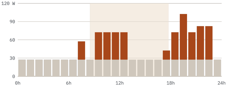
Figura 1.1. Consumo medio, hora a hora, en un día de invierno. Gris: el suelo constante de frigorífico, rúter e inversor; naranja: todo lo demás; banda clara: horas de luz.
