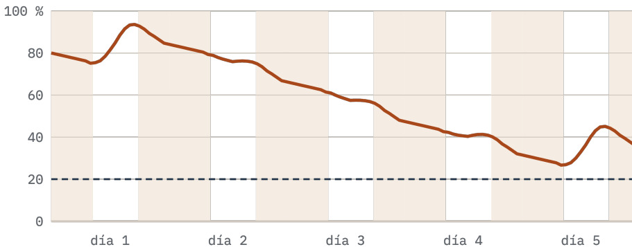
Figura 3.1. Estado de carga del banco de 5,1 kWh durante cinco días de diciembre: despejado, tres nublados, despejado. Sombreado: noche. Discontinua: el suelo del 20 %.
