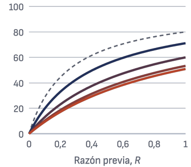
Figura 1. VPP (probabilidad de que un resultado de la investigación sea verdadero) en función de la razón de probabilidades previa al estudio para varios niveles de sesgo, u
