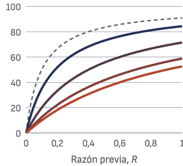
Figura 1. VPP (probabilidad de que un resultado de la investigación sea verdadero) en función de la razón de probabilidades previa al estudio para varios niveles de sesgo, u
