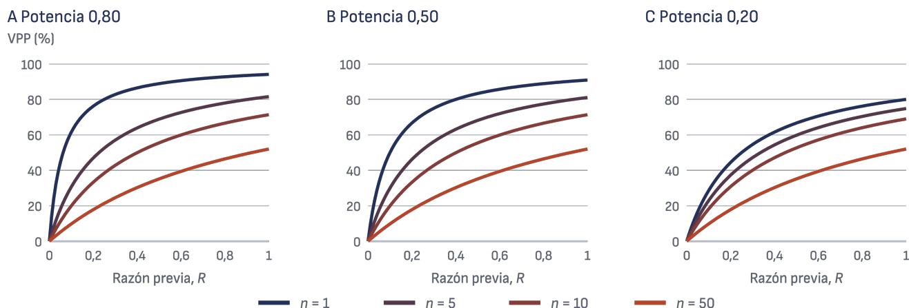
Figura 2. VPP (probabilidad de que un resultado de la investigación sea verdadero) en función de la razón de probabilidades previa al estudio para distintos números de estudios, n
