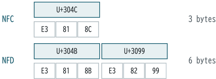
図 3-1 「が」の二つの表し方。上段が符号位置、下段が UTF-8 のバイト列
