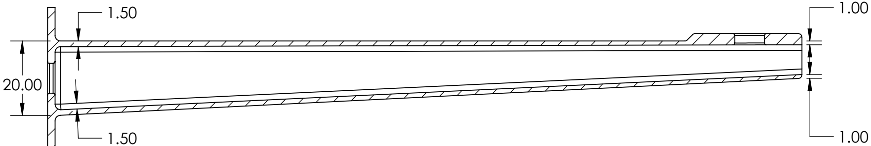
SECTION A-A
