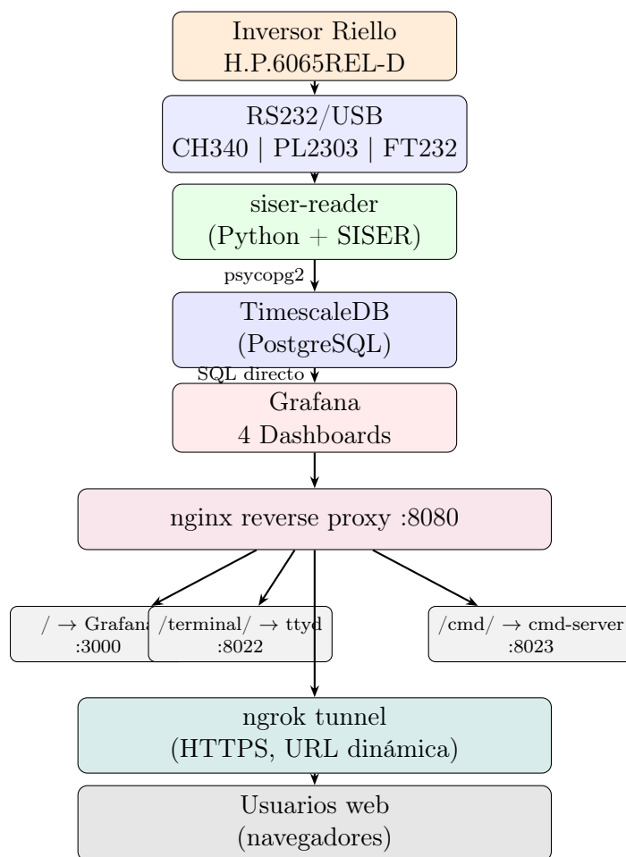
Figura 1: Arquitectura general del sistema de monitoreo
