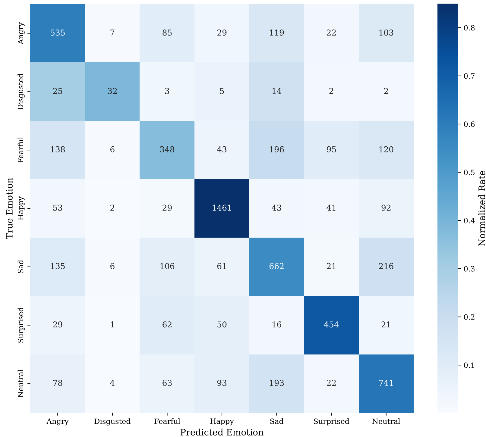
Confusion Matrix: FER
