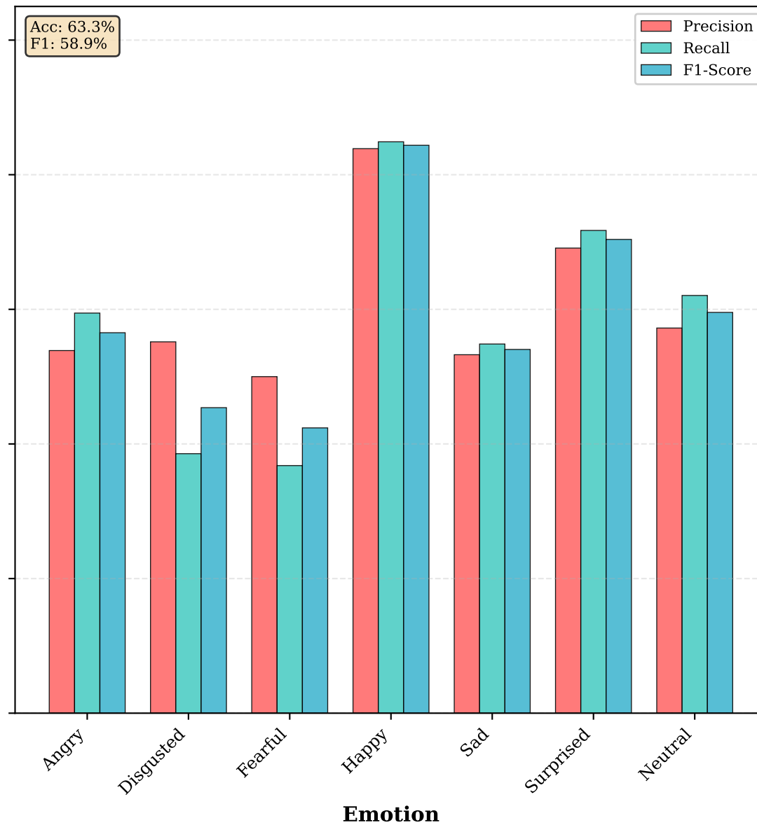
FER
