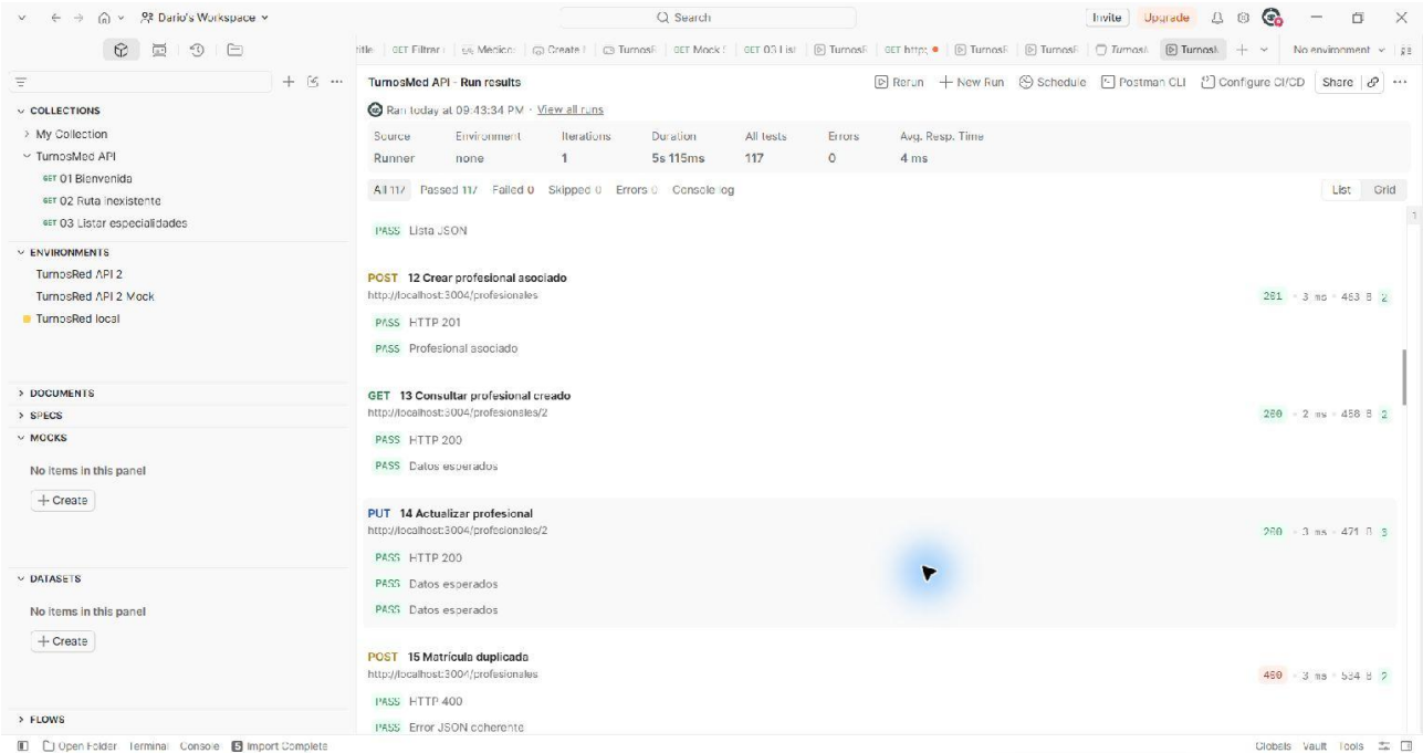
Figura 4. Ejecución real: 117 pruebas aprobadas, 0 fallidas, 0 omitidas y 0 errores; Environment none. Las URLs resueltas usan localhost:3004.
