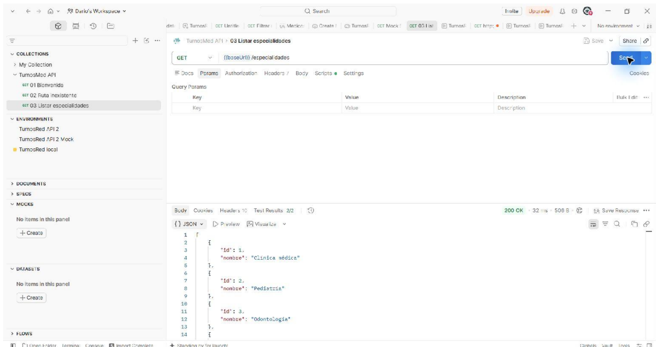
Figura 3. Petición con {{baseUrl}}/especialidades , respuesta 200 OK y Test Results 2/2.
