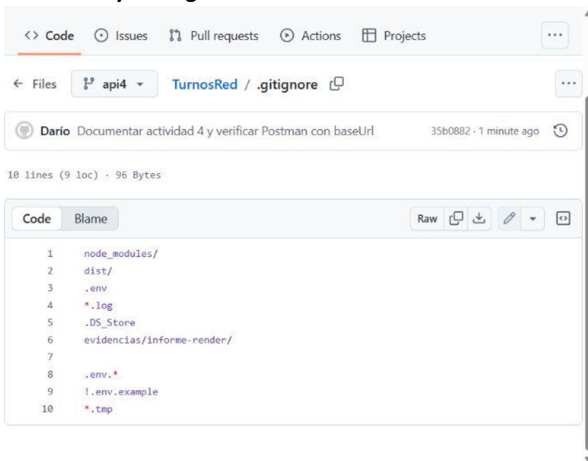
Figura 9. .gitignore publicado: exclusión de node_modules/, dist/ y .env. .env.example se conserva como plantilla sin secretos.
