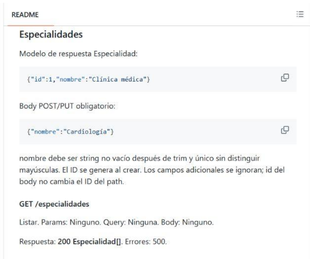
Figura 5. Modelo JSON, body de entrada y documentación de GET /especialidades.
