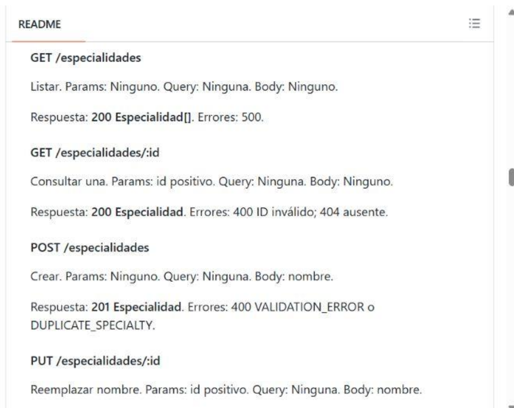
Figura 6. Referencia de GET, GET por ID y POST de Especialidades. El README continúa con las demás operaciones.
