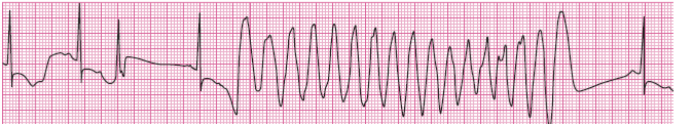
FIGURA 1.13A: TORSADES DE POINTES (TAQUICARDIA VENTRICULAR POLIMORFA)
