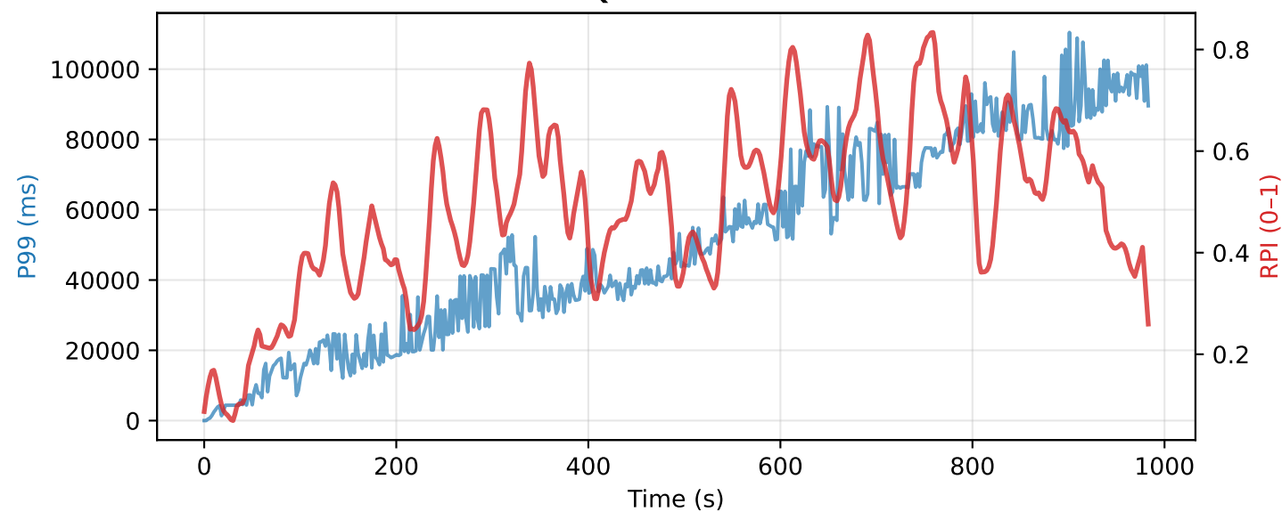
EMQX: P99 & RPI
