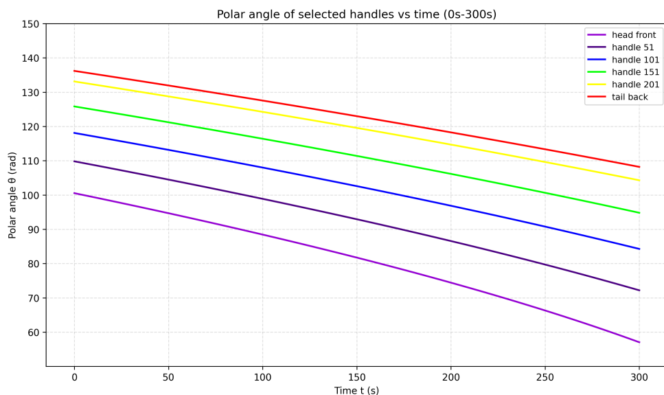
图 4: 问题一代表性把手极角随时间变化
