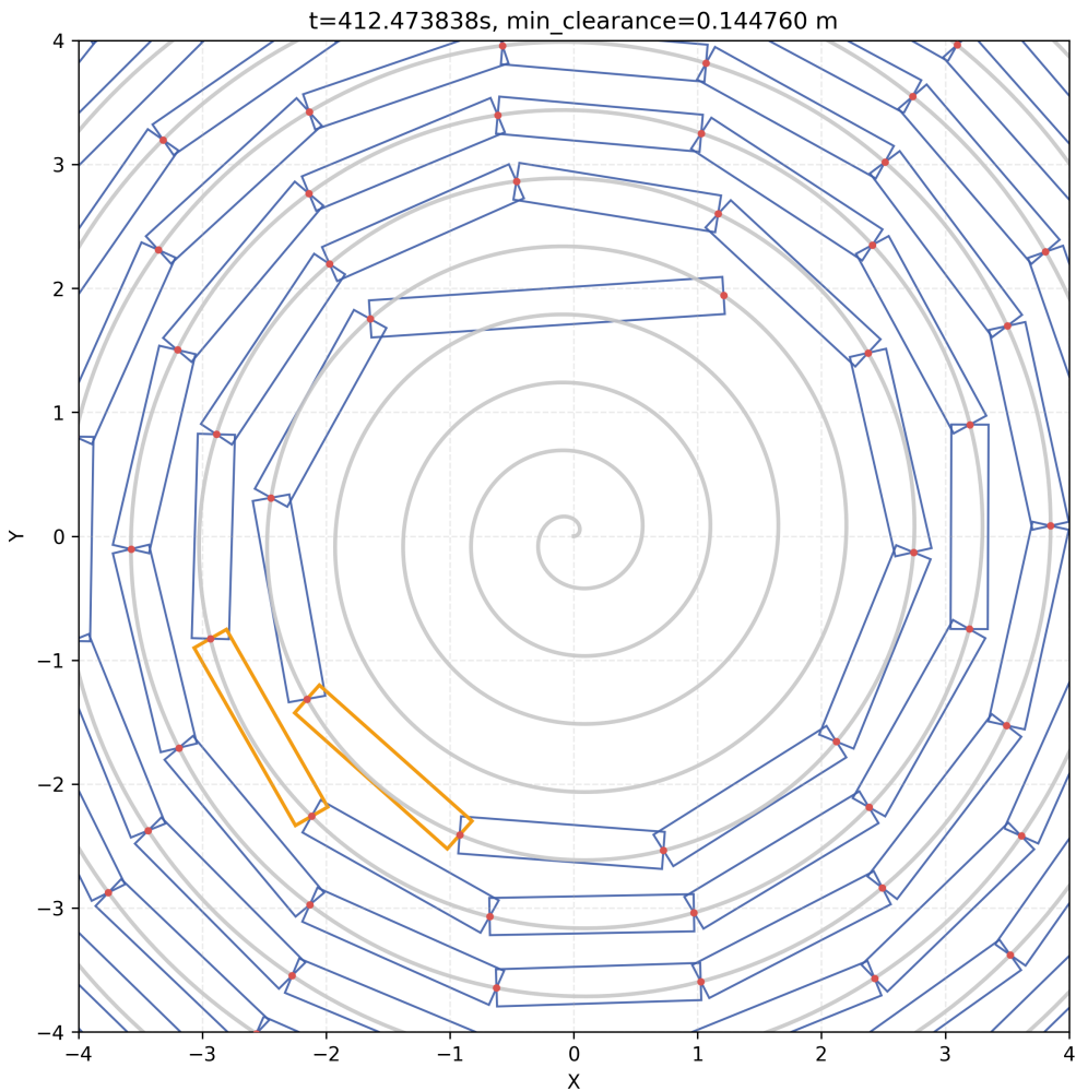
图 7: 问题二首次碰撞附近的整队构型
