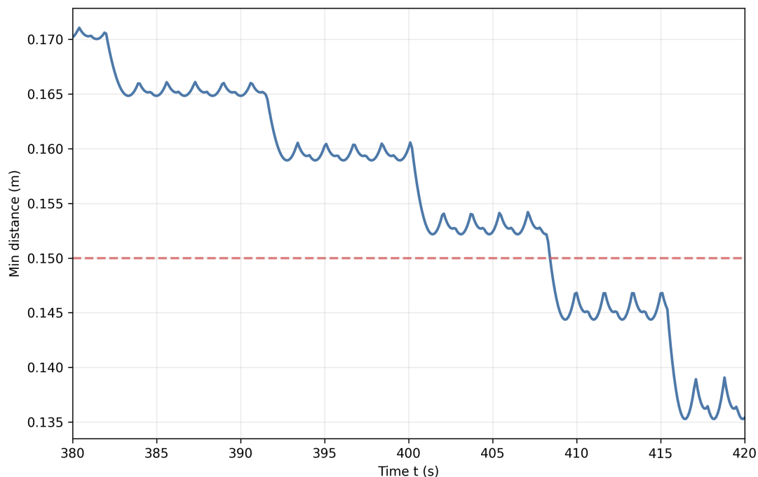
图 8: 问题二最小距离随时间变化曲线
