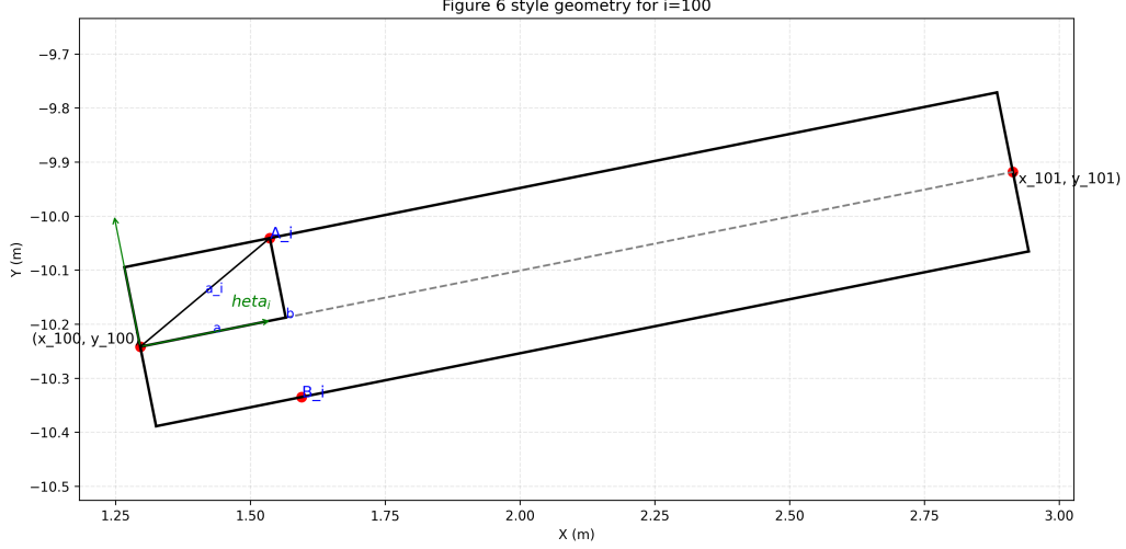
图 6: 问题二单节板凳几何抽象示意
