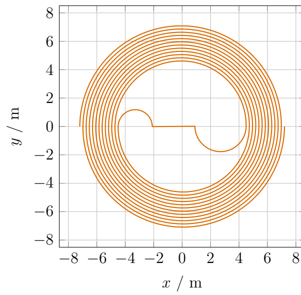
图 11: 问题四调头路径
