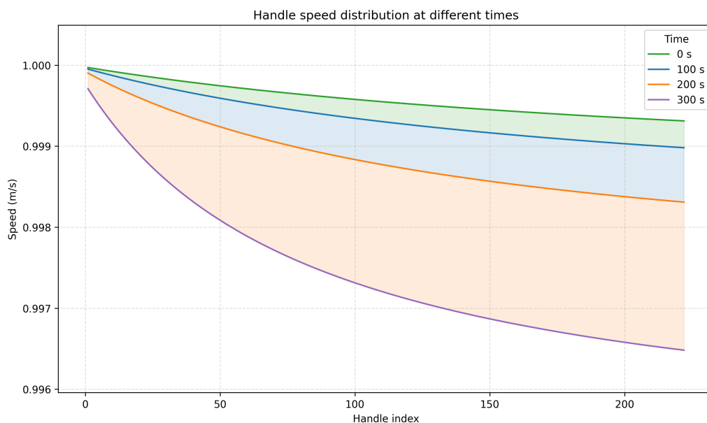
图 5: 问题一不同时间下的把手速度分布
