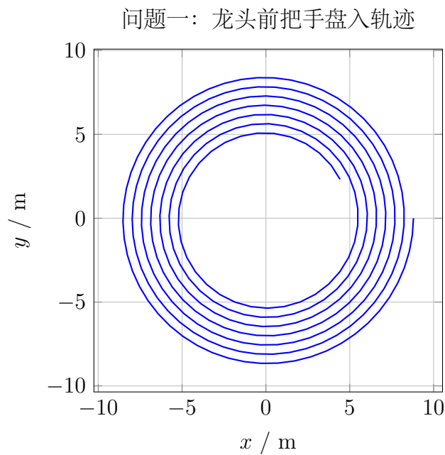
图 2: 问题一龙头前把手完整轨迹
