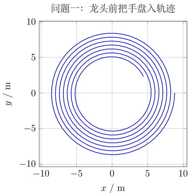
图 2: 问题一龙头前把手完整轨迹
