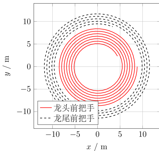
图 3: 问题一关键把手轨迹对比
