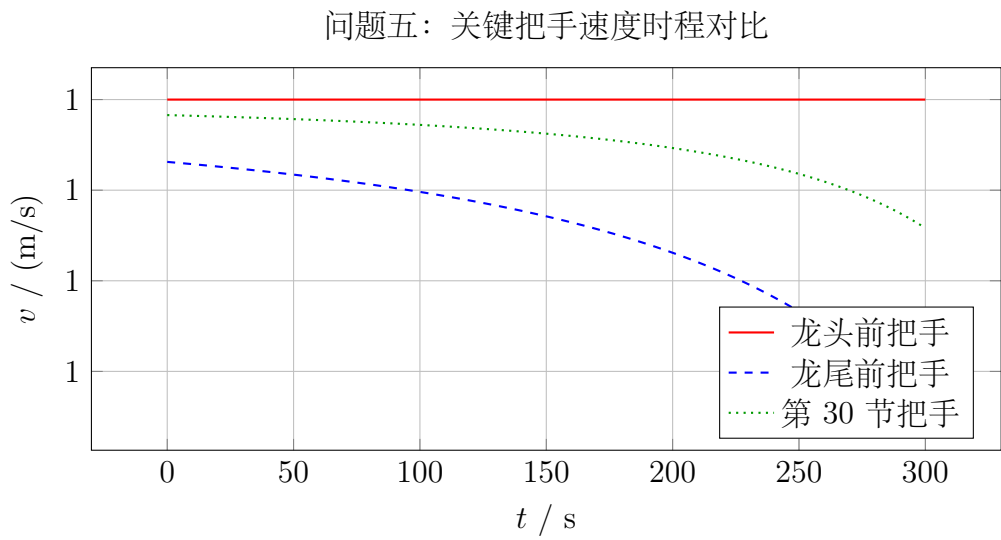
图 11: 问题五关键把手速度对比
