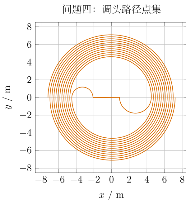
图 8: 问题四调头路径
