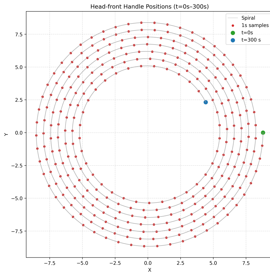
图 12: 问题一龙头前把手位置散点补充图
