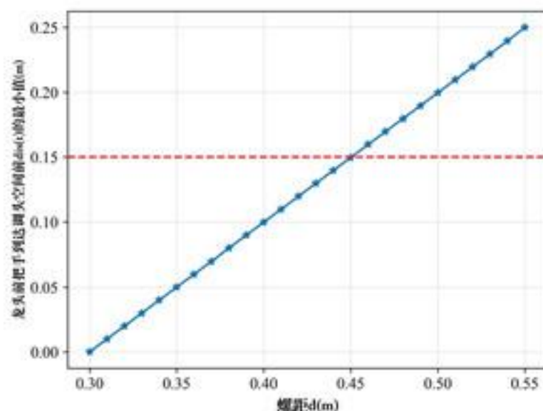
图15 dis(t) 最小值随螺距 d 变化图像
