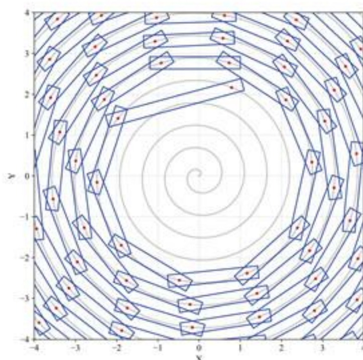
图8 停止盘入时刻板凳龙碰撞情况
