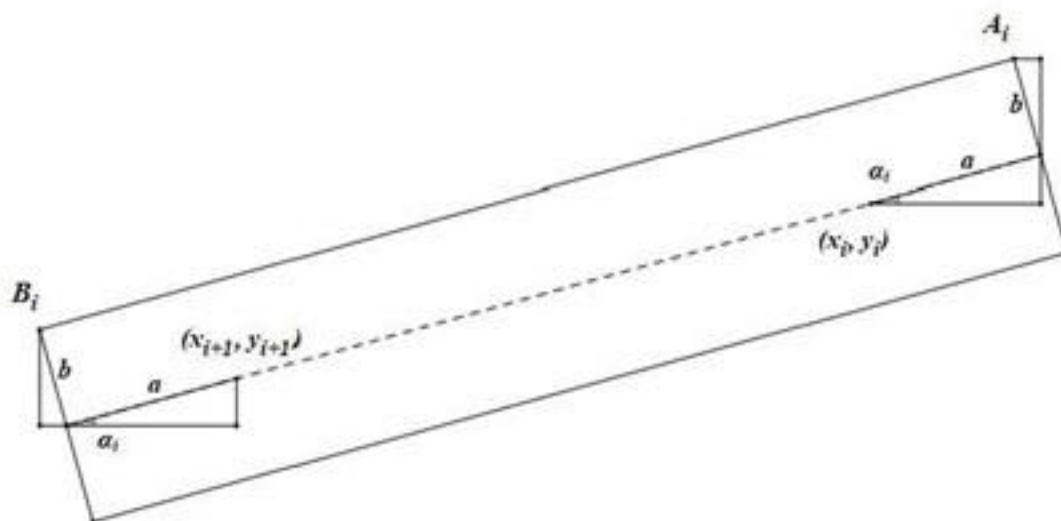
图6 编号为 i 的板凳几何关系示意图
