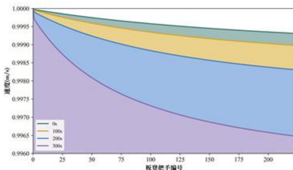
图 4 不同时刻下板凳龙把手的速度情况
