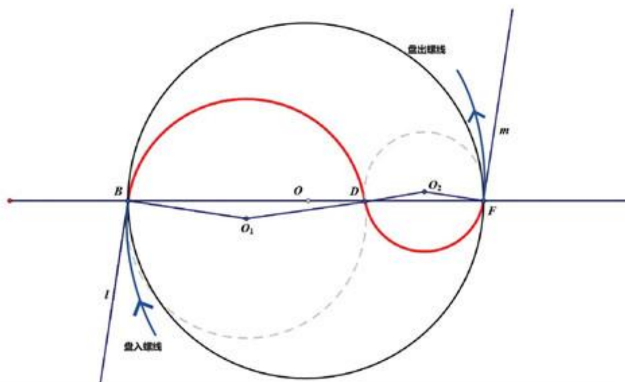
图 16 调头曲线示意图
