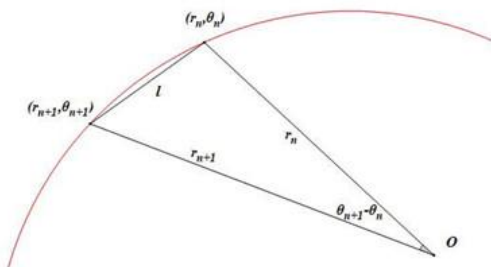
图 2 相邻把手几何关系示意图
