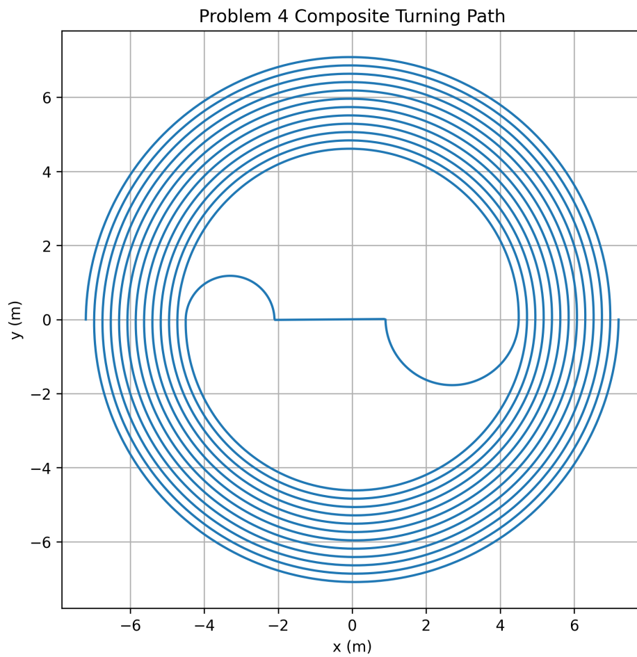
图 16: 问题四路径总览（程序原始输出图，作为补充）
