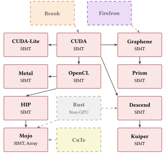
Fig. 23. Descendants of CUDA [239].
