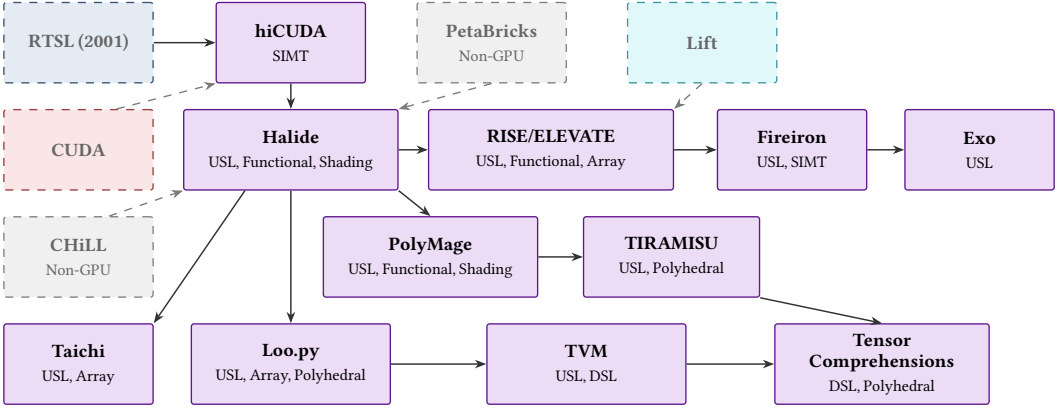
Fig. 32. Descendants of Halide [288, 289].
