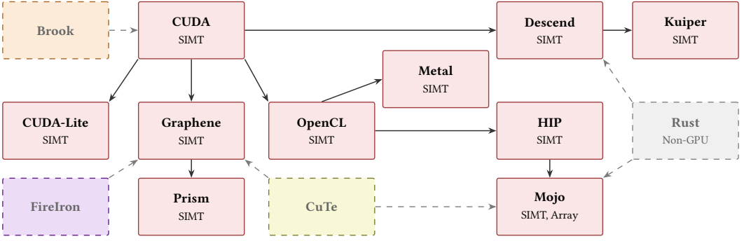
Fig. 23. Descendants of CUDA [239].
