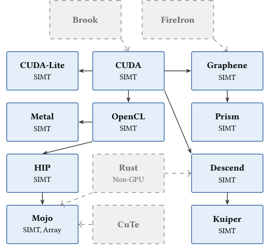
Fig. 23. Descendants of CUDA [232].
