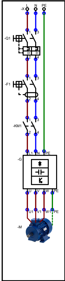
Circuito de potencia
