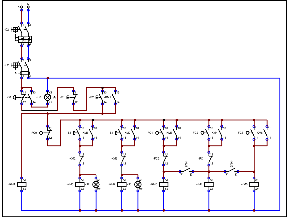
Circuito de mando
