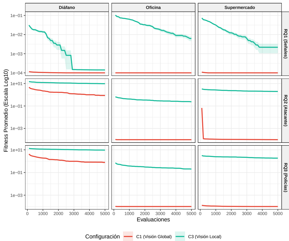
Figure 1: Evolución de fitness promediada (30 ejecuciones, 5 simulaciones por evaluación) para C1 (Visión Global) y C3 (Visión Local).
