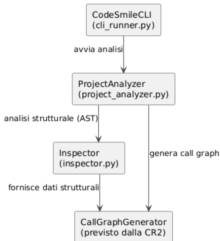
Fig. 3 – CR2: Call graph concettuale utilizzato per l’Impact Analysis.
