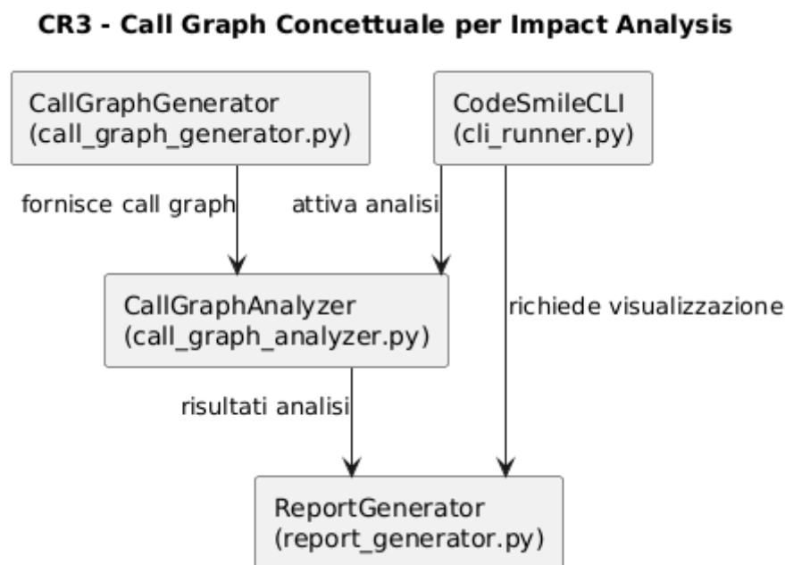
Fig 5. – CR3: Call graph concettuale utilizzato per la dependency-based impact analysis.
