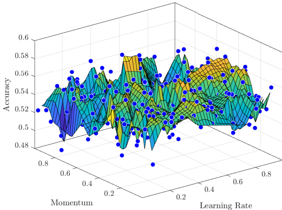
Nesterov Momentum
