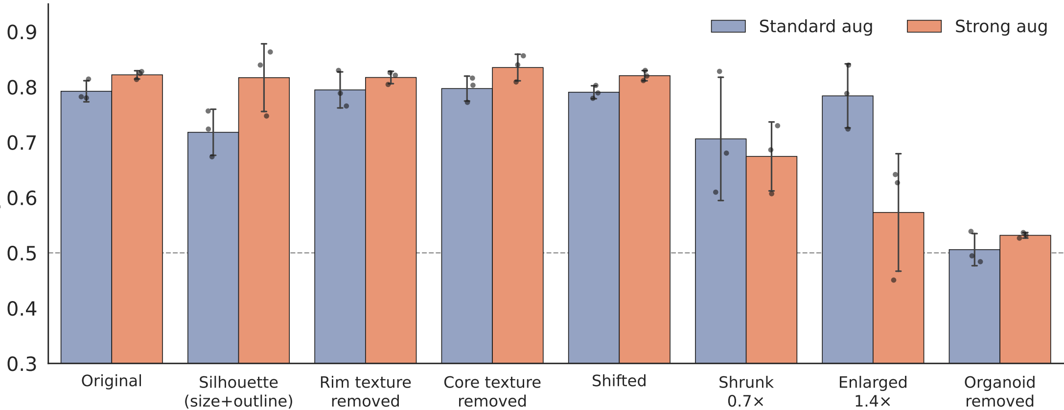
AUC (days 24/28/30)
