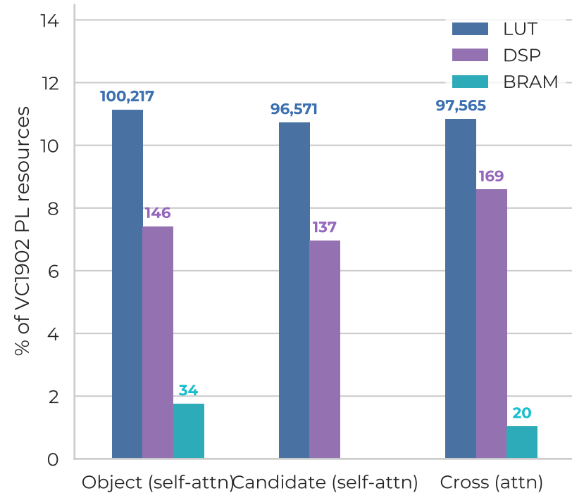
PL utilization per block
