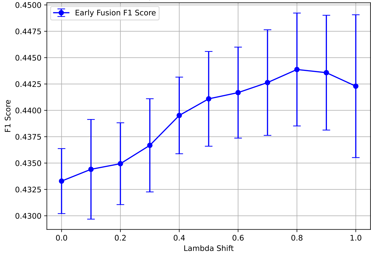
Early Fusion F1 Score - ham10000
