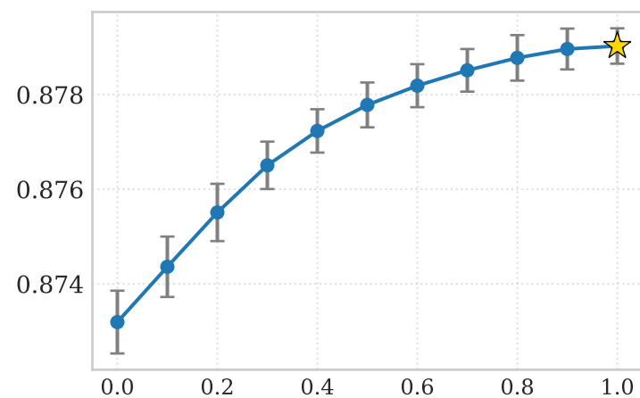
BRSET AUC
