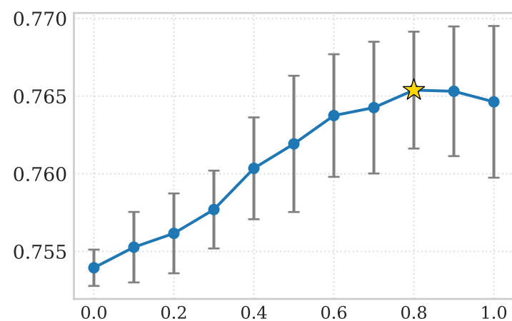
HAM10000 AUC
