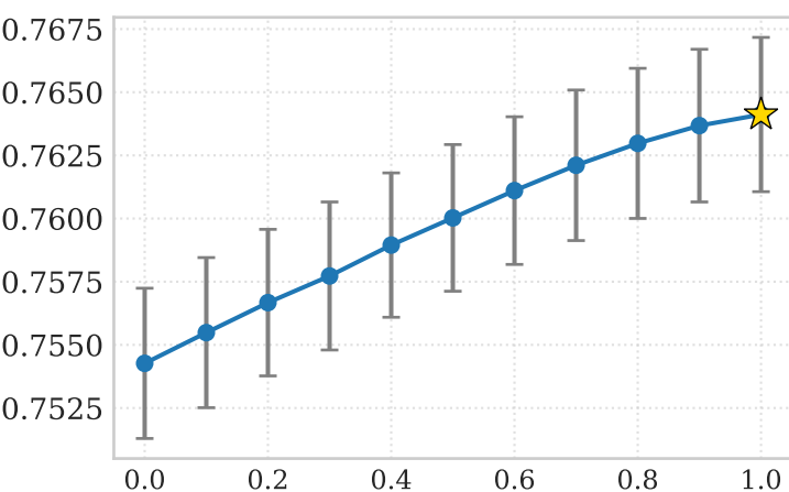
mBRSET AUC
