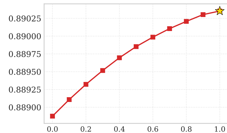
MedSigLIP (Medical)
