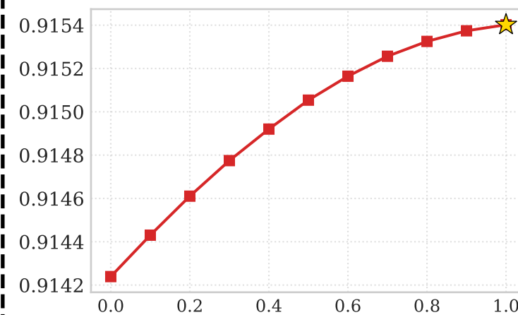
BioMedCLIP (Medical)
