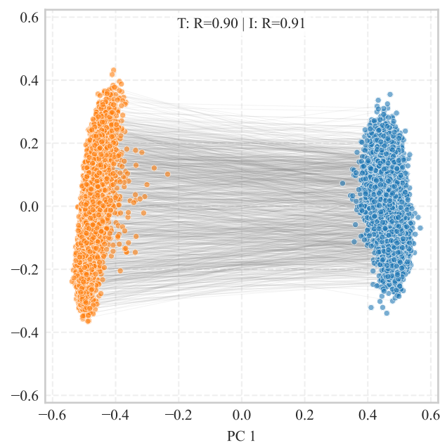
BioMedCLIP (Medical)
