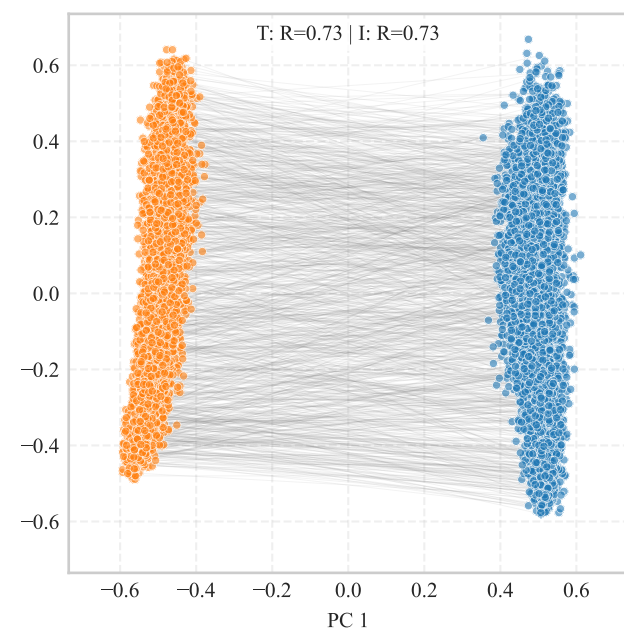
MedSigLIP (Medical)
