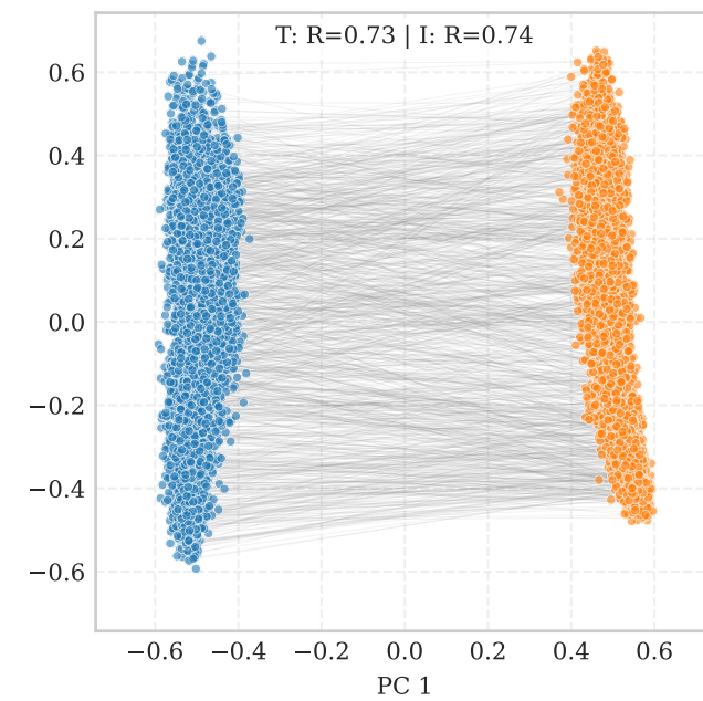
MedSigLIP (Medical)
