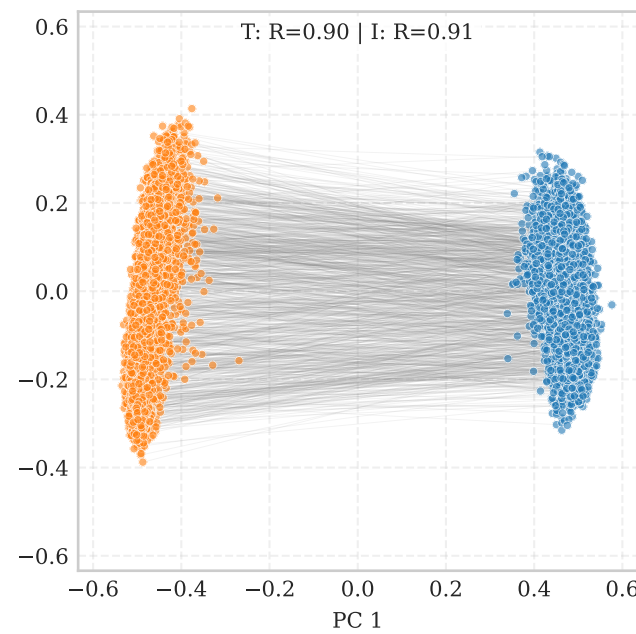
BioMedCLIP (Medical)
