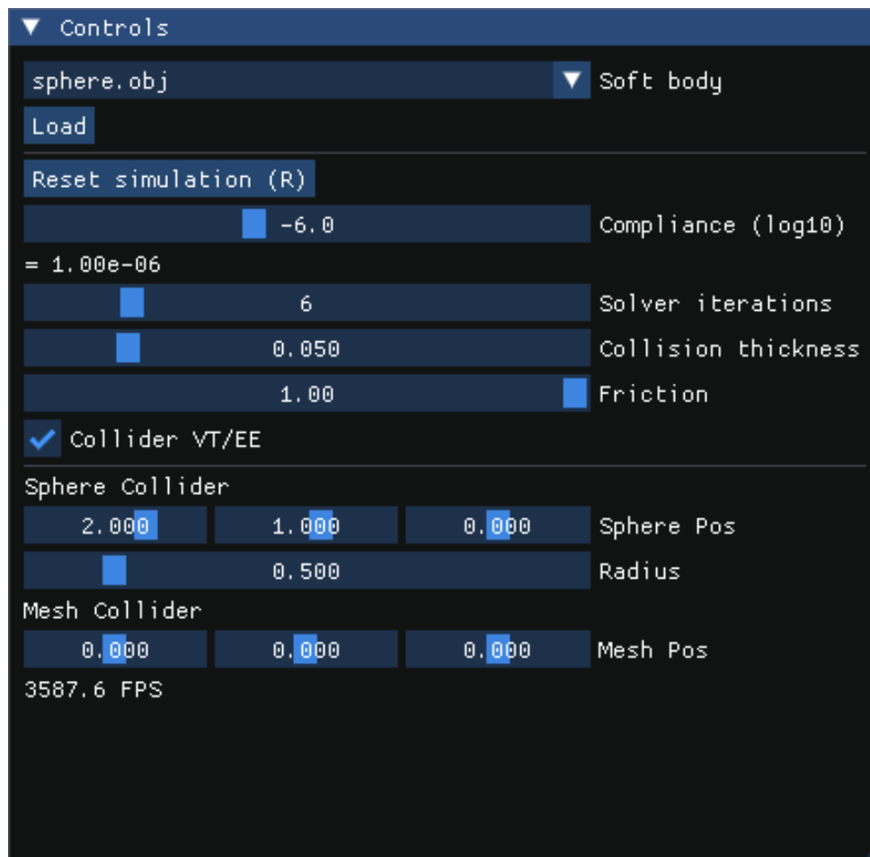
Слика 7.2: Слика од корисничкиот интерфејс
