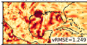
b) Linear error
