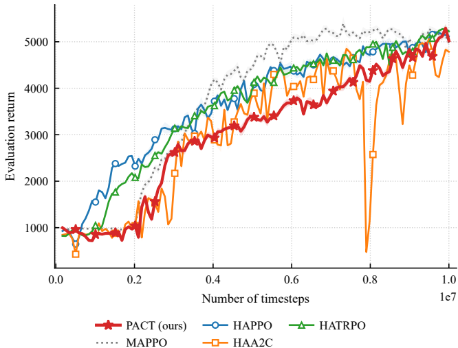
MAMuJoCo Ant-v2 4x2
