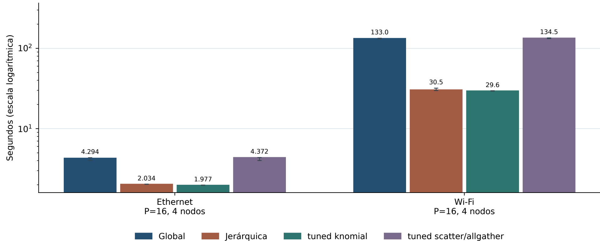
Difusión aislada de B (75.5 MB), 16 procesos en 4 nodos
