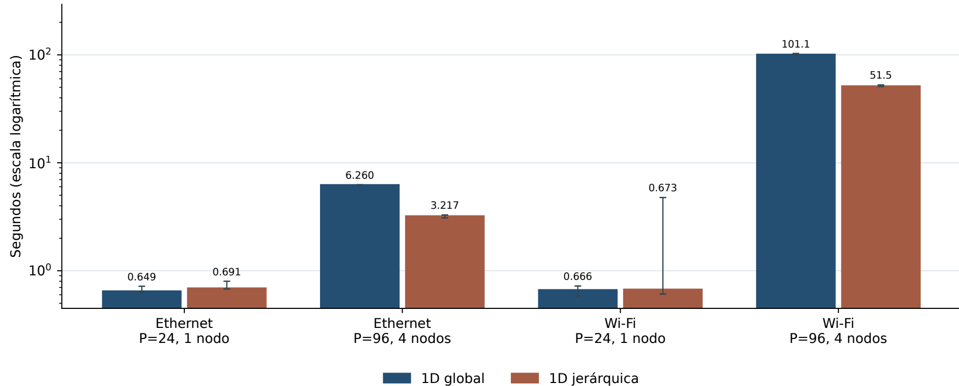
Multiplicación completa, N=3072 (mediana, mínimo y máximo)
