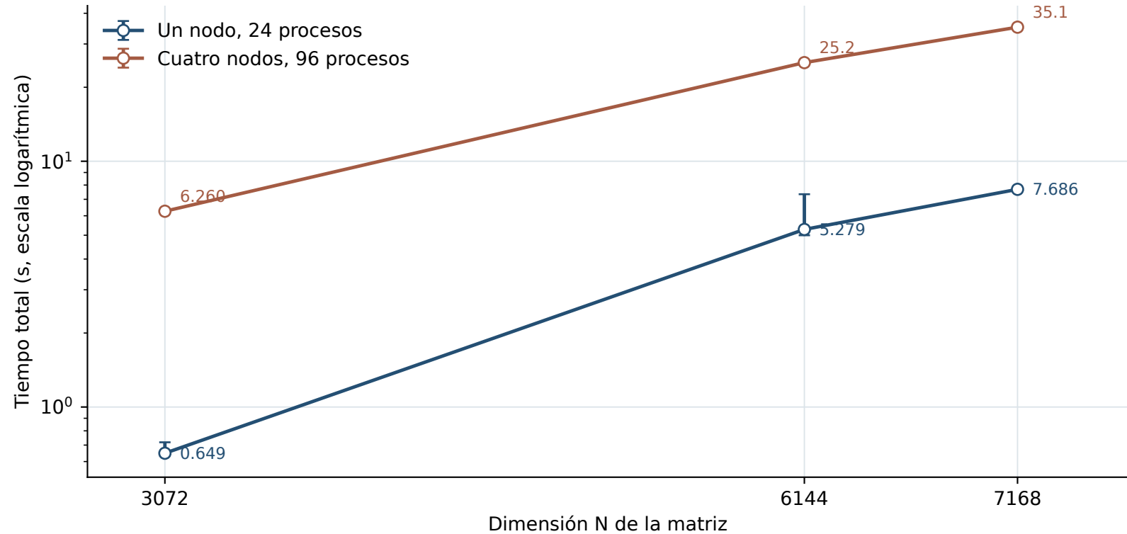
Escalamiento por tamaño en Ethernet (1D global)
