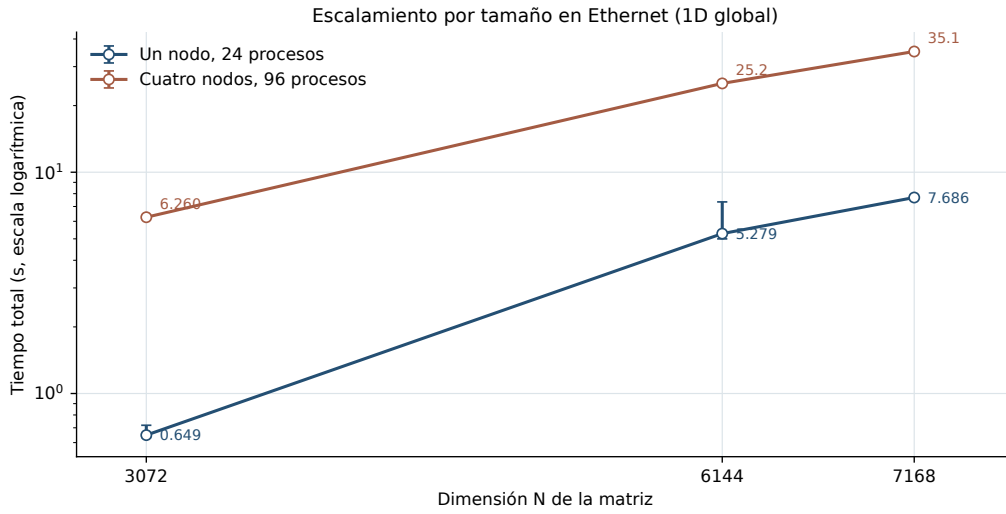
Figura 6: 1D global por Ethernet. Medianas con mínimo y máximo: cinco repeticiones para N = 3072 y tres para N = 6144, 7168 .
