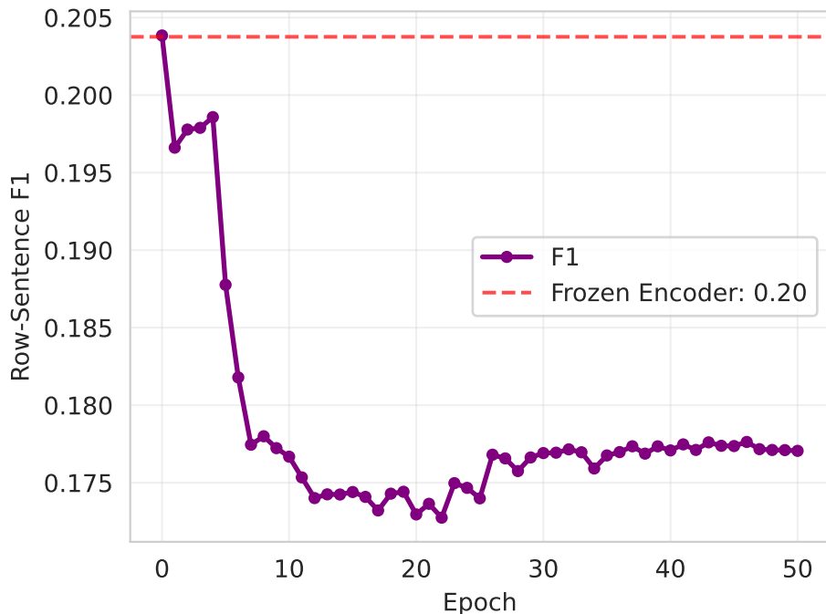
Row-Sentence F1
