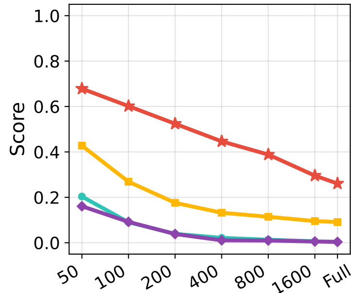
F1@8
