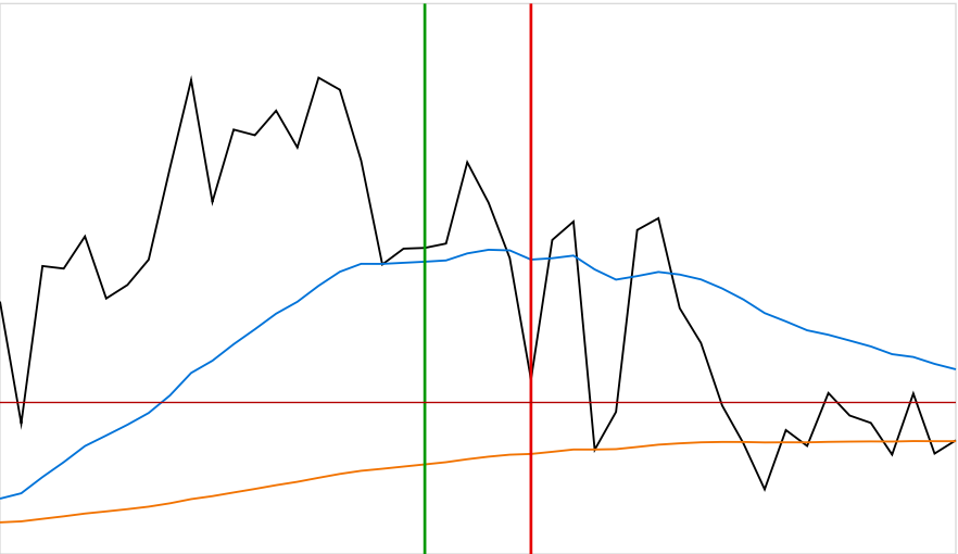
ENTRY_A_STOP_B_EXIT_B_TEMPORAL_TEST_0003
