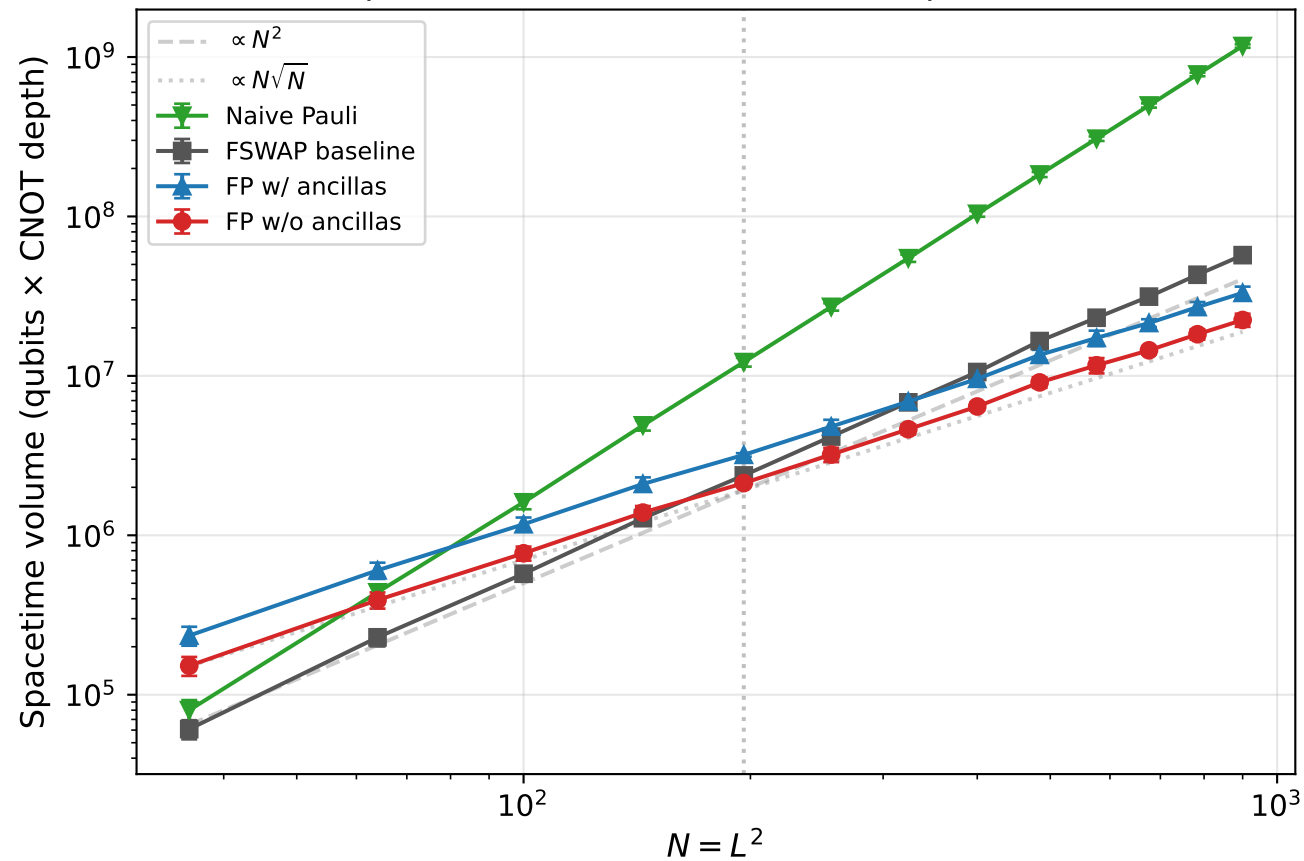
Spacetime Volume Per Trotter Step (k=1.0)
