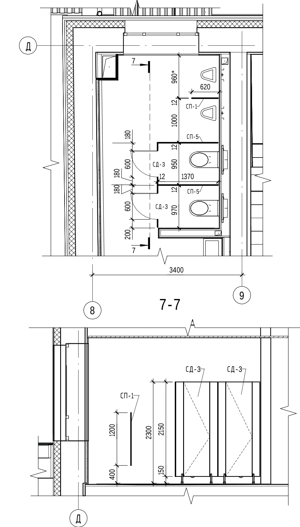
Сантехнические перегородки в помещении 213
