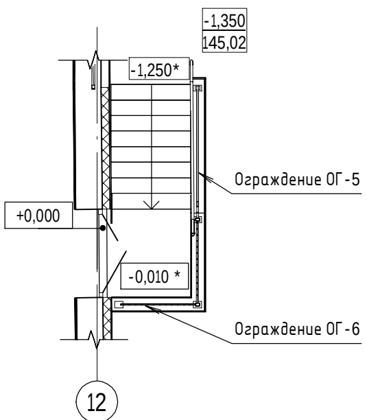
План 1-го этажа (Крыльцо №2 по оси 12)
