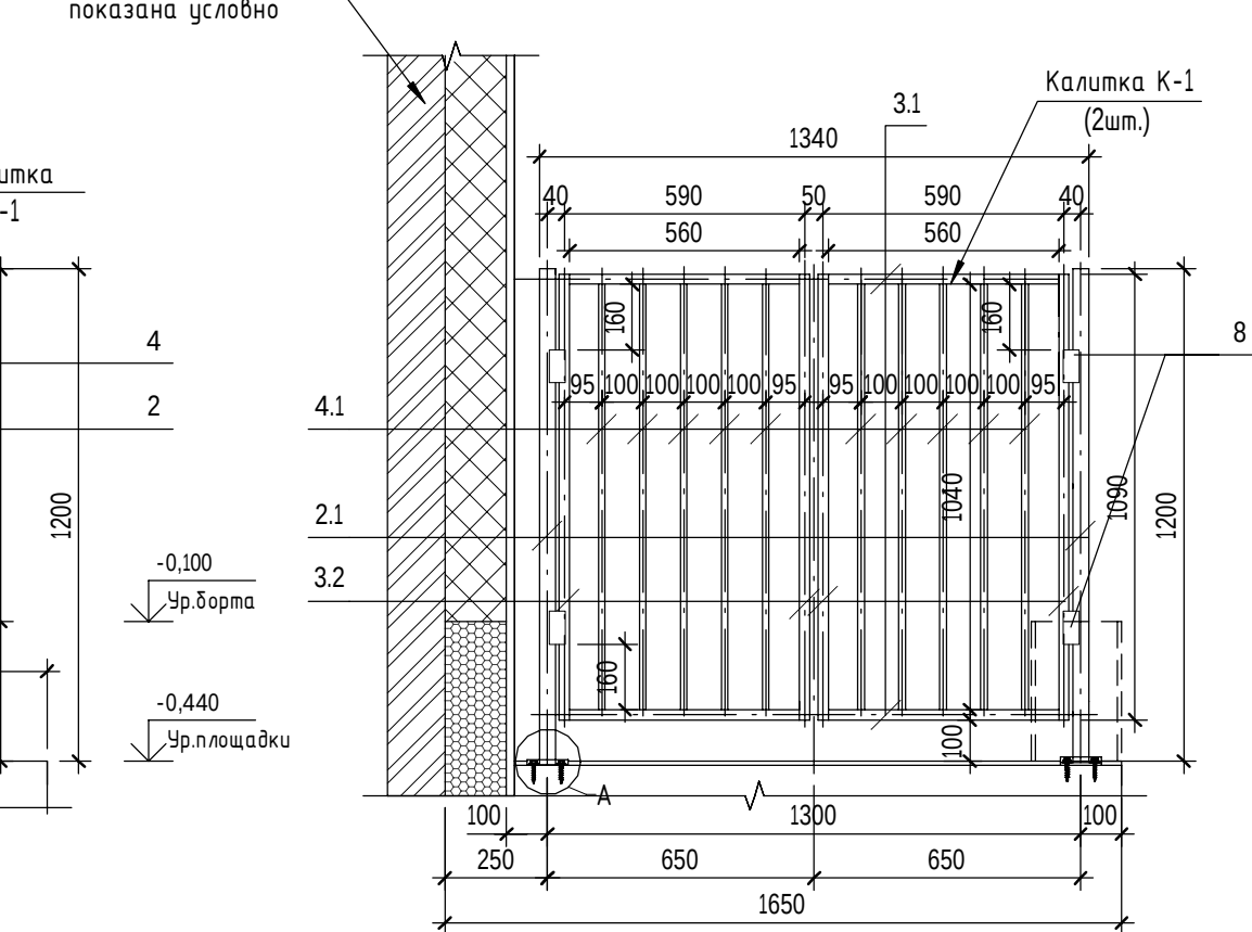
Распашная калитка К-1
