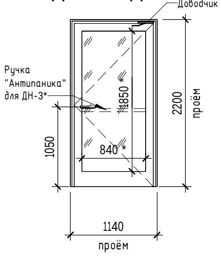
ДН-3н/ДН-3*
