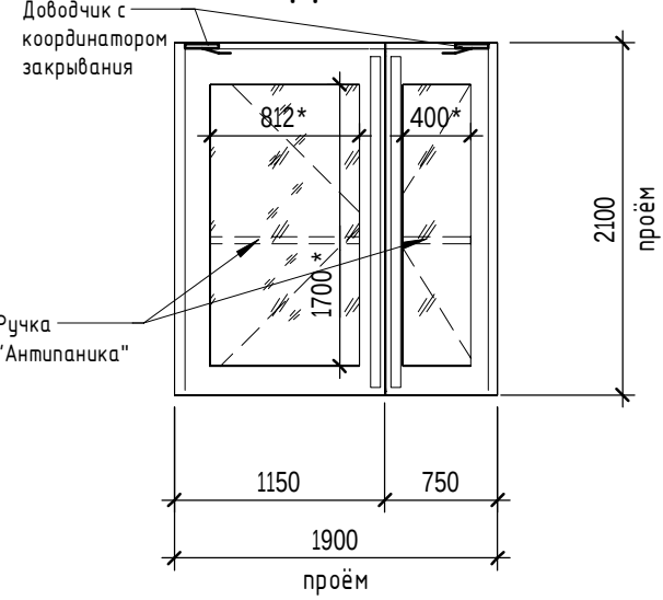
ДН-4н
