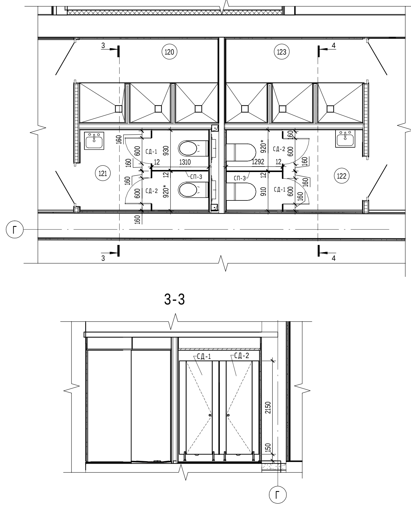
Сантехнические перегородки в помещении 120, 121, 122, 123
