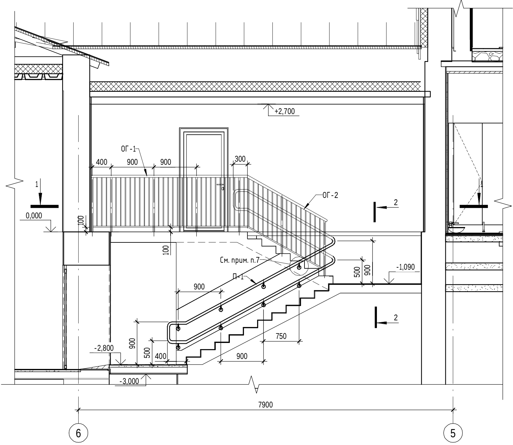
Лестница в осях 5-6/Г-Д
