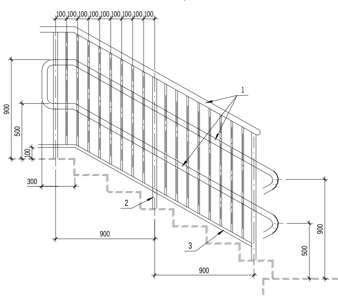
Ограждение ОГ-2
