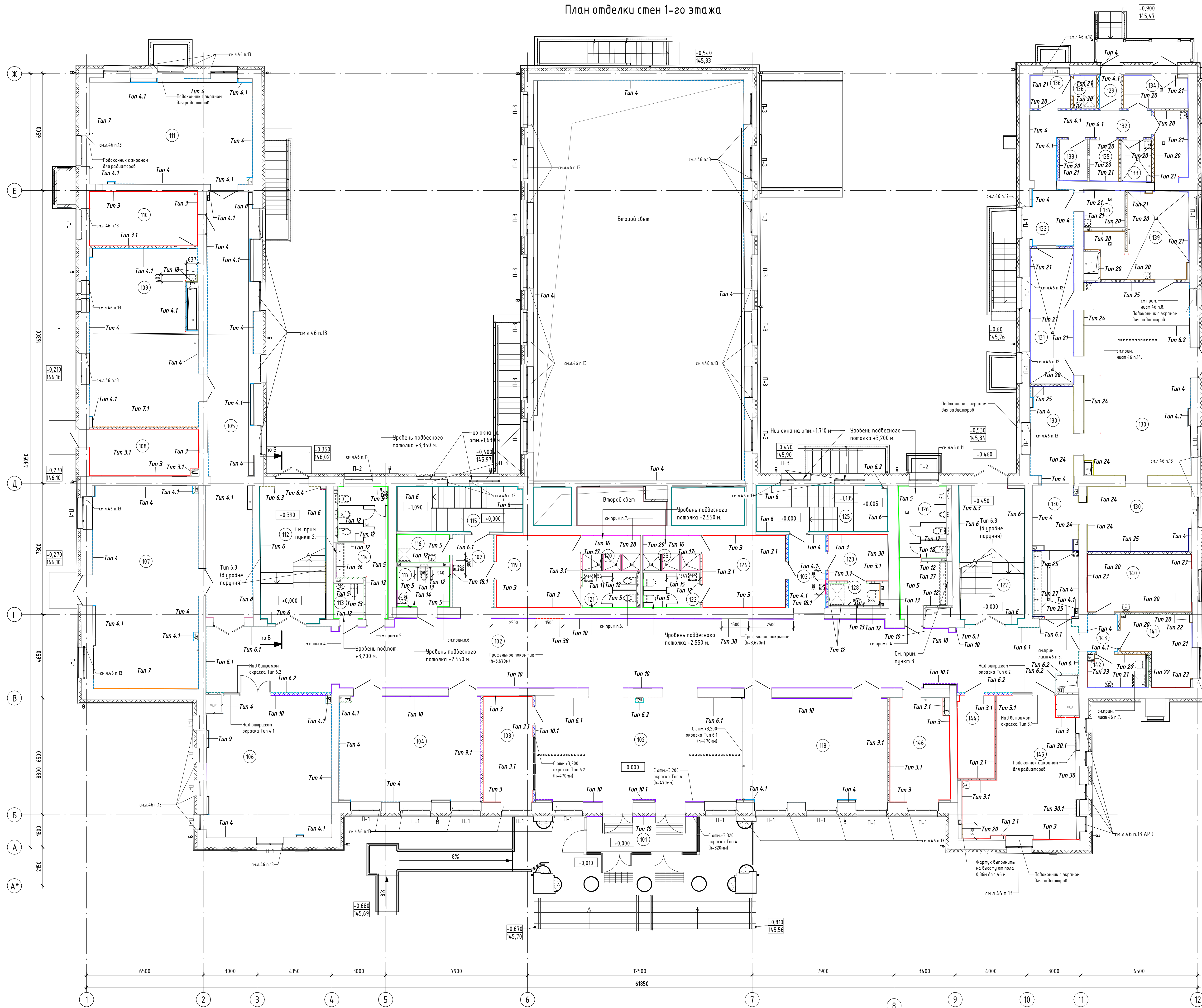
План отделки стен 1-го этажа
