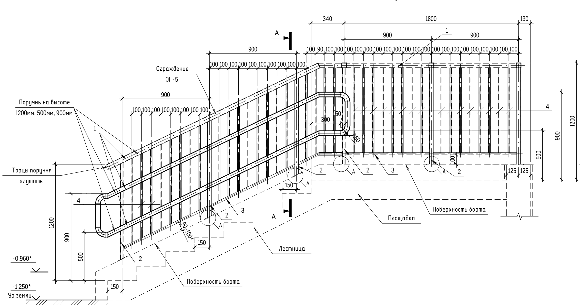
Ограждение ОГ-5
