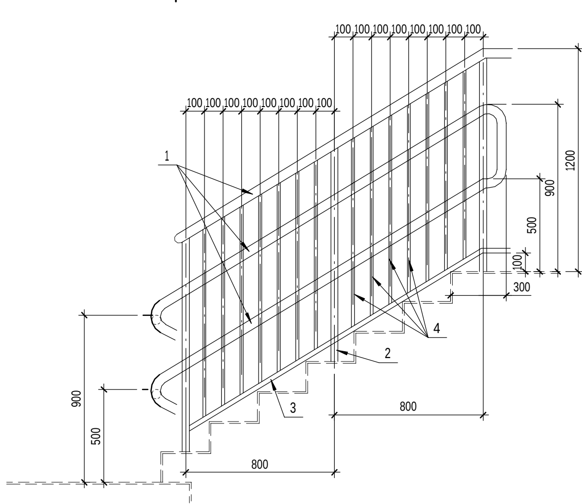
Ограждение ОГ-4
