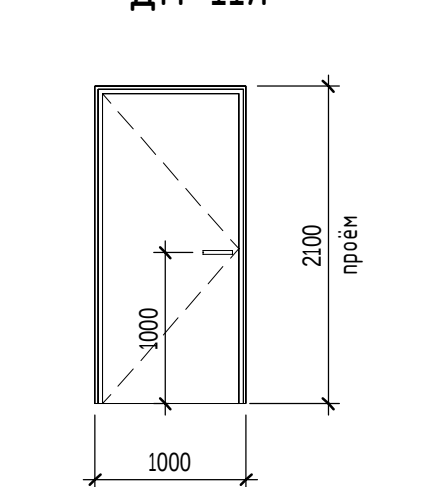
ДН-11л
