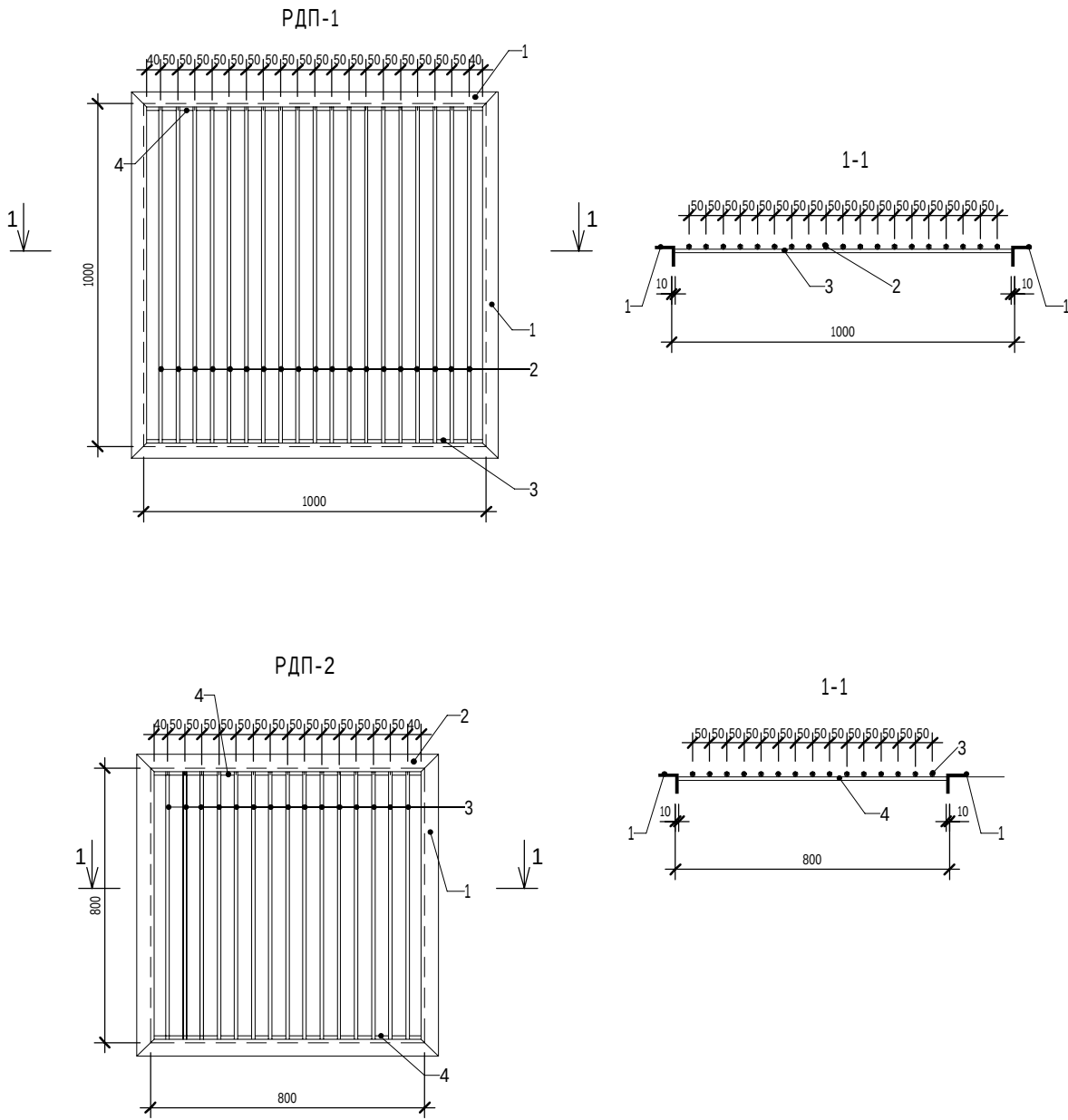
Металлическая решётка для прямка
