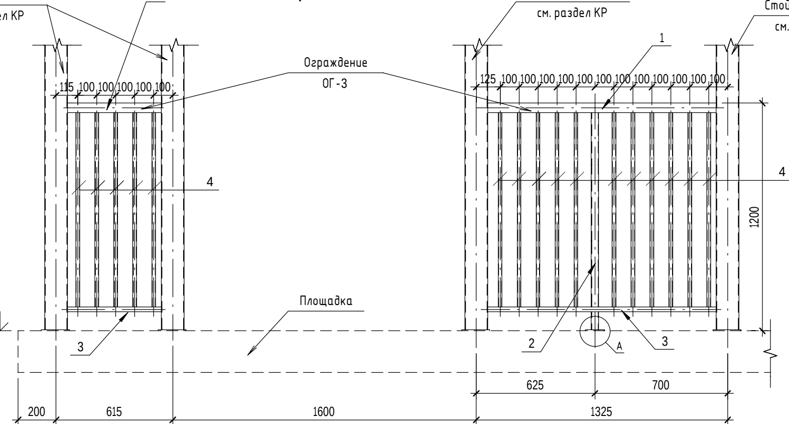
Ограждение ОГ-3
