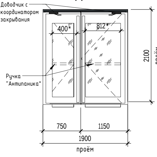
ДН-4л
