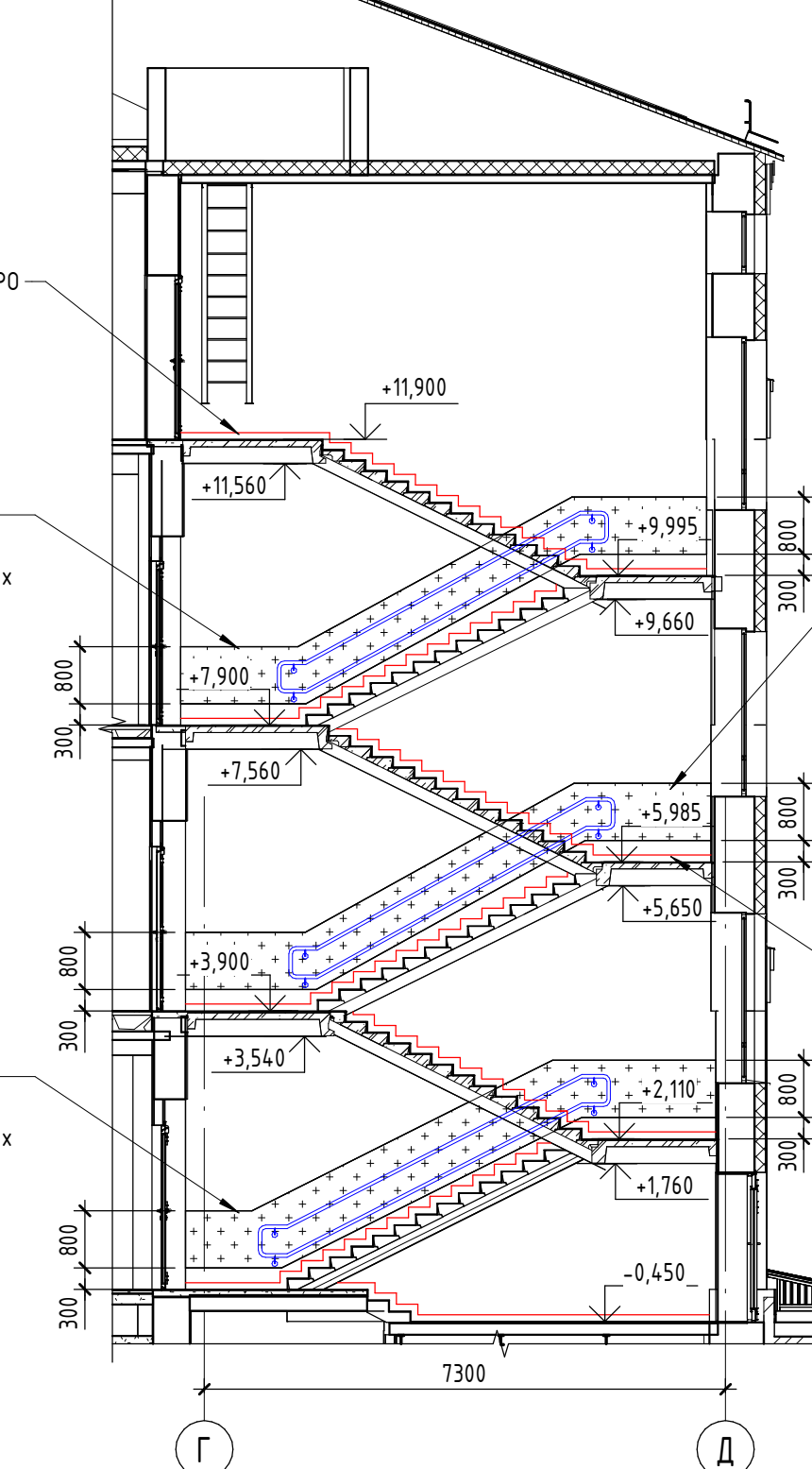
Б-Б по лестнице в осях 9-10/Г-Д
