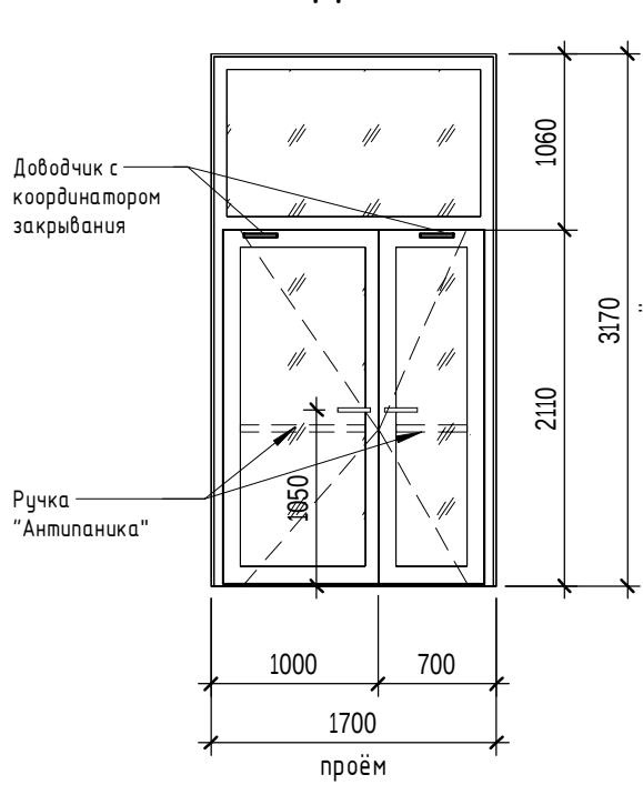
ДН-1л
