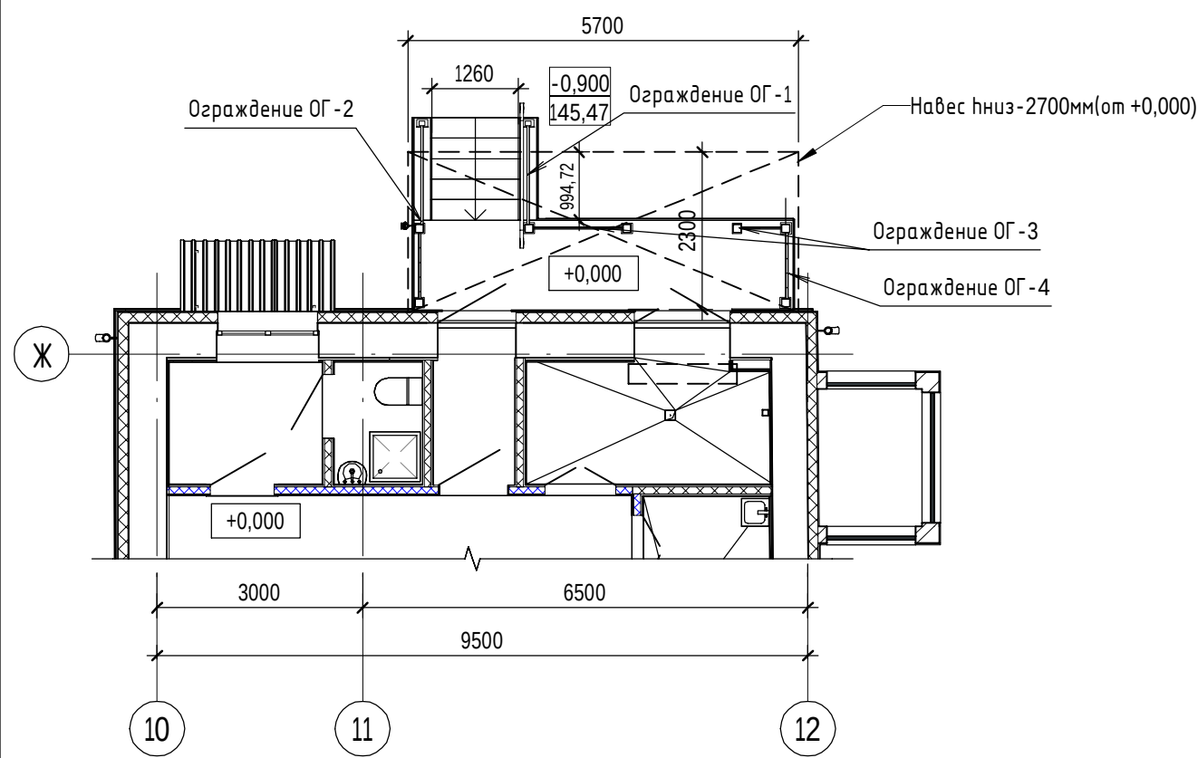
Ограждение ОГ-1
