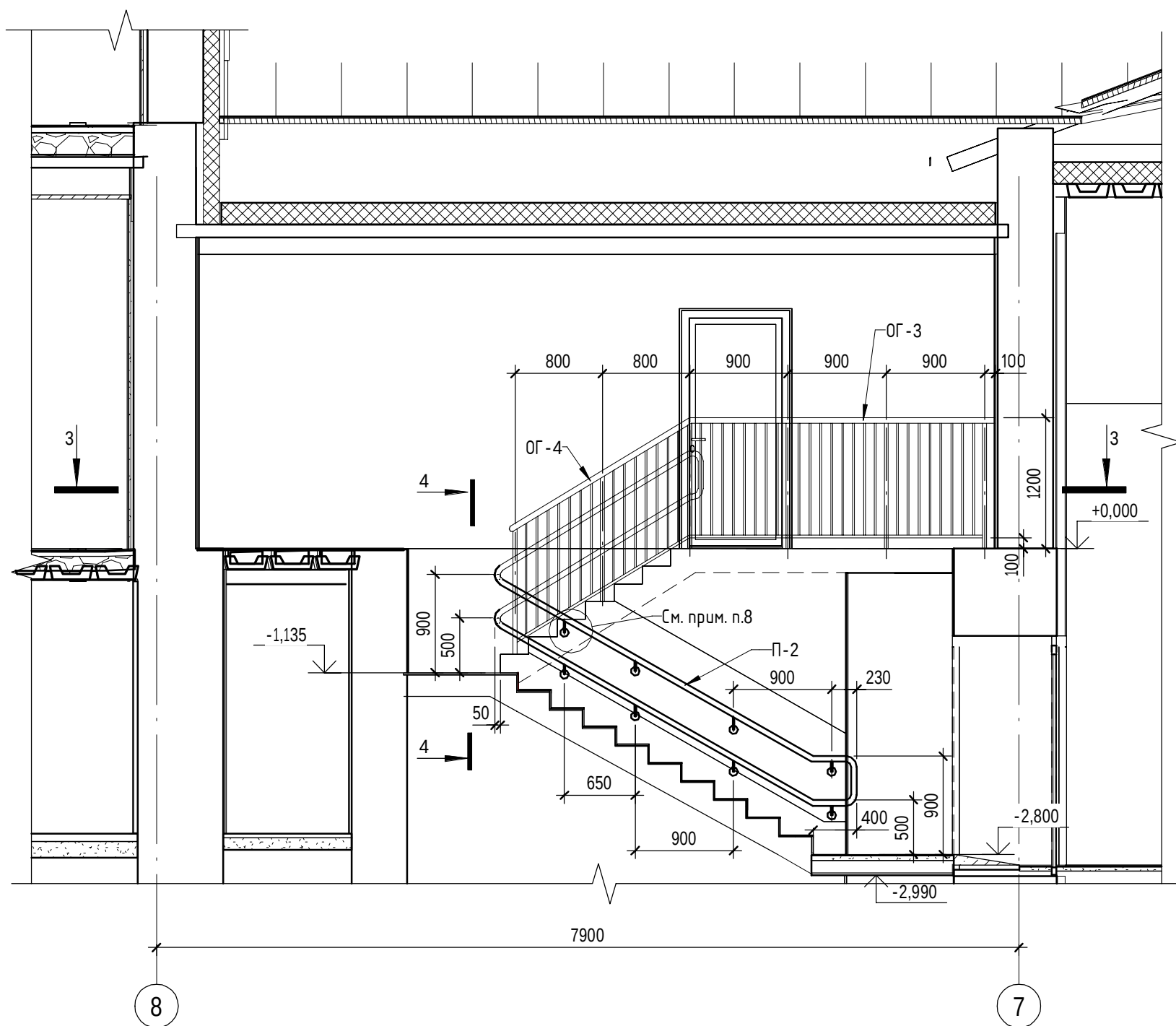
Лестница в осях 7-8 /Г-Д
