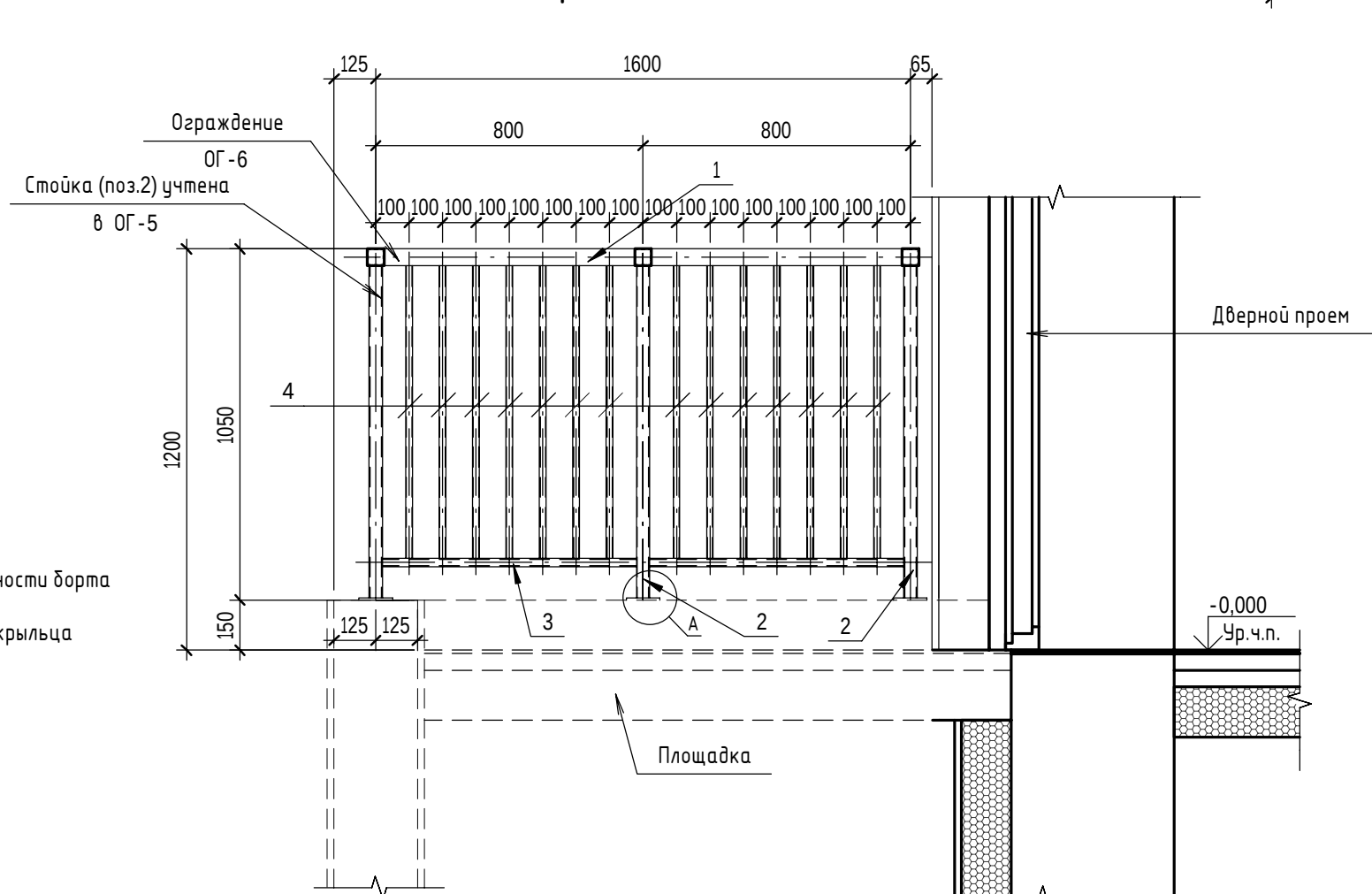
Ограждение ОГ-6
