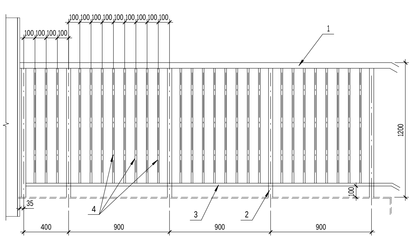
Ограждение ОГ-1
