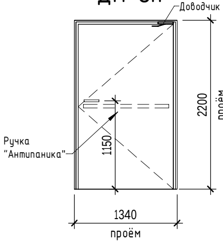
ДН-8н
