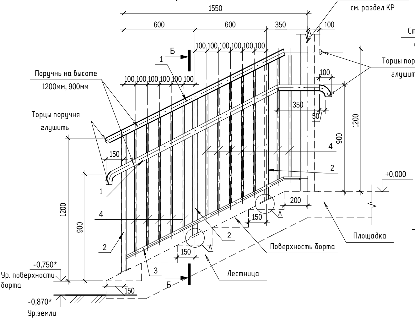
Ограждение ОГ-1
