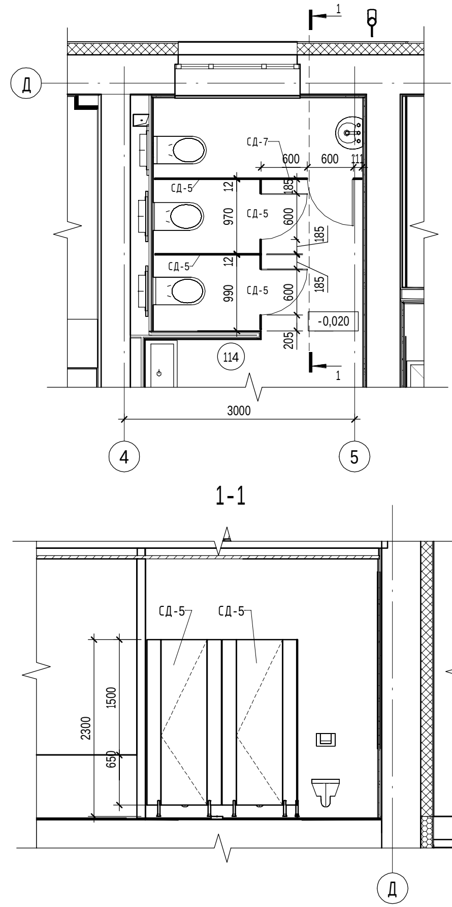
Сантехнические перегородки в помещении 114
