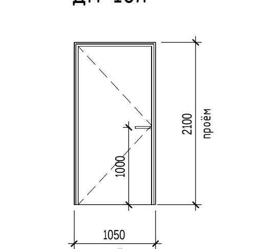
ДН-10л
