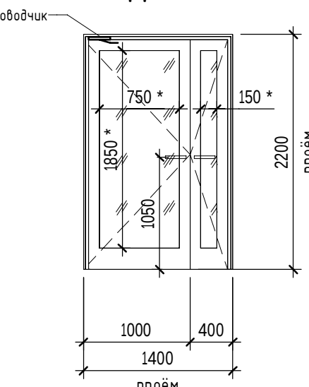
ДН-2л
