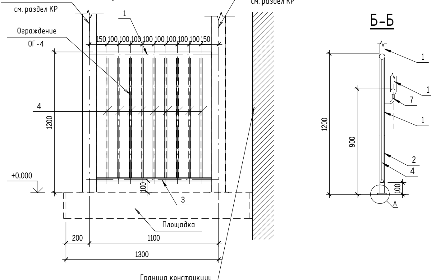
Ограждение ОГ-4
