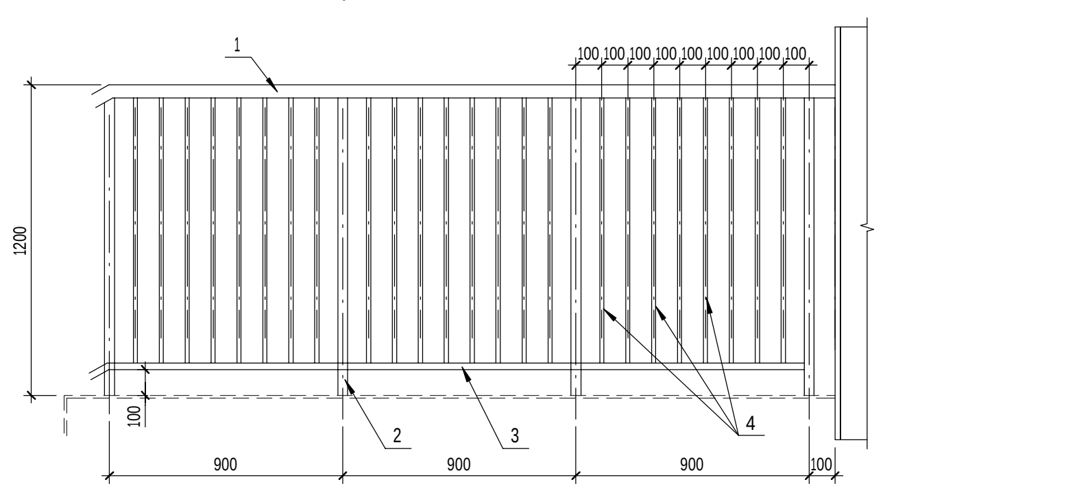
Ограждение ОГ-3
