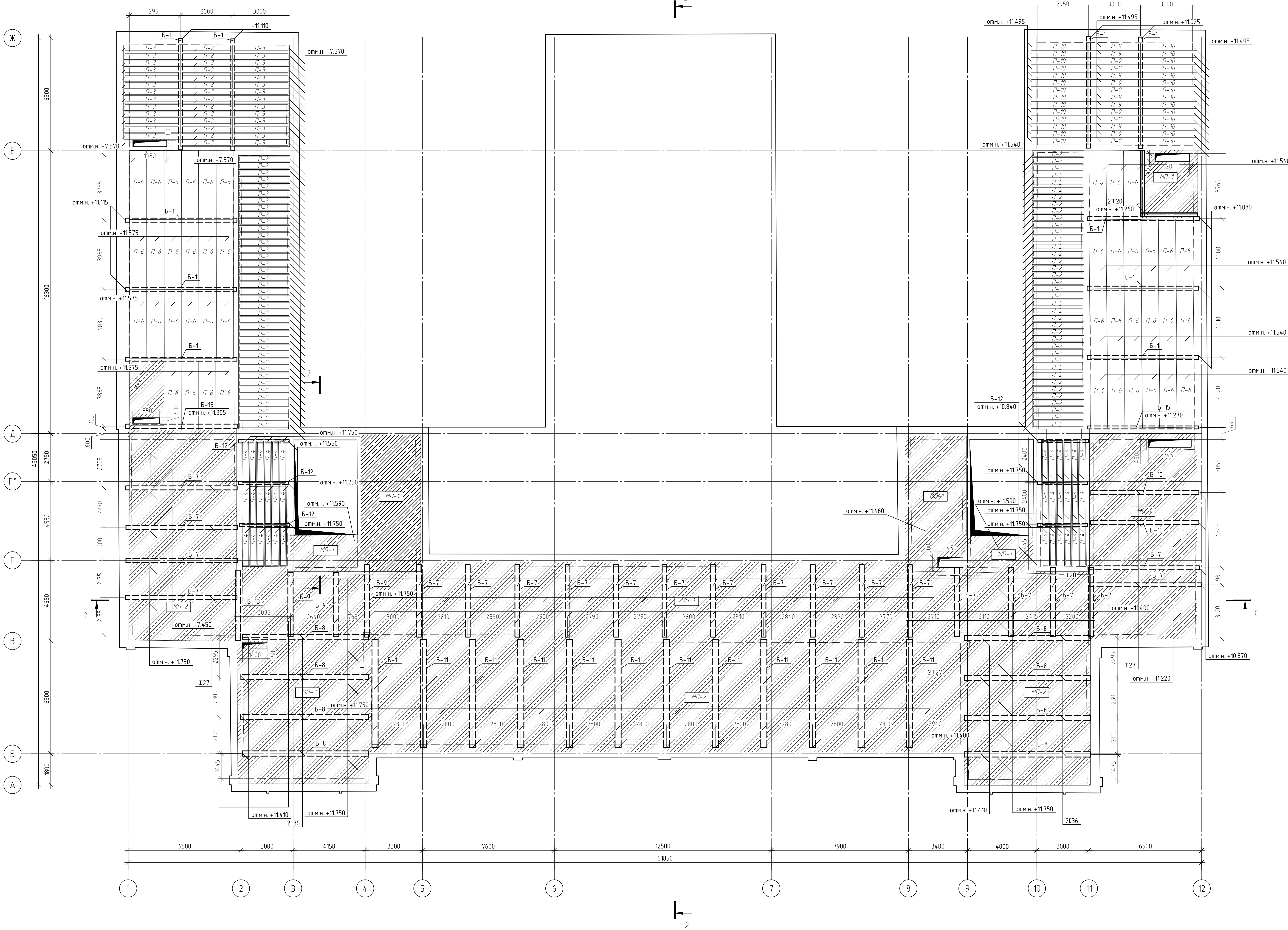
План перекрытия 3-го этажа
