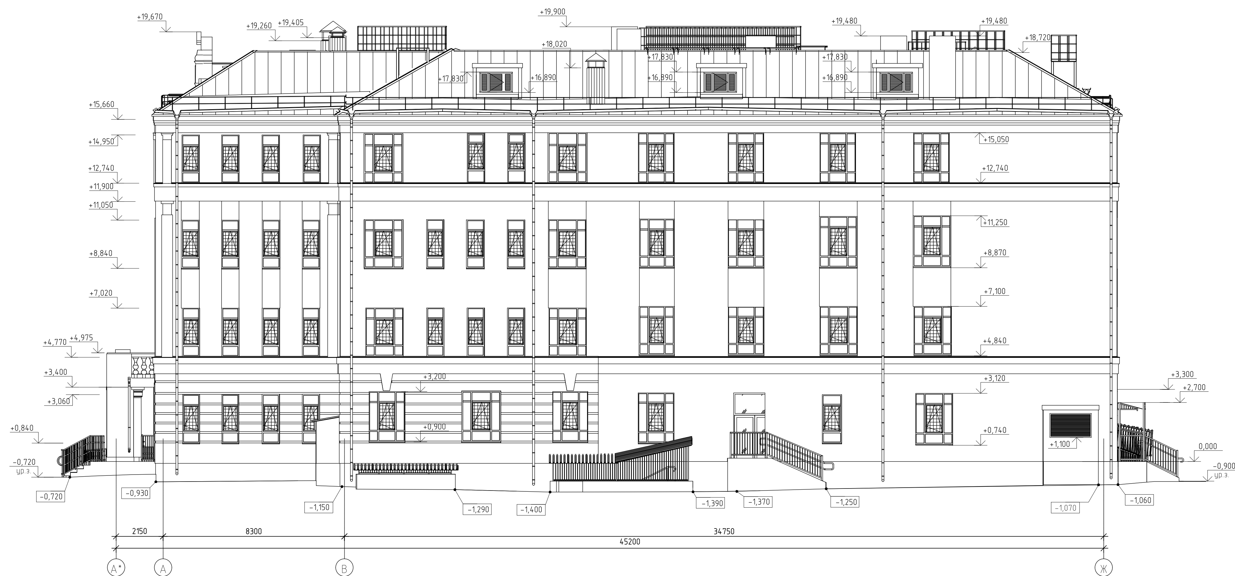
Фасад в осях А*-Ж
