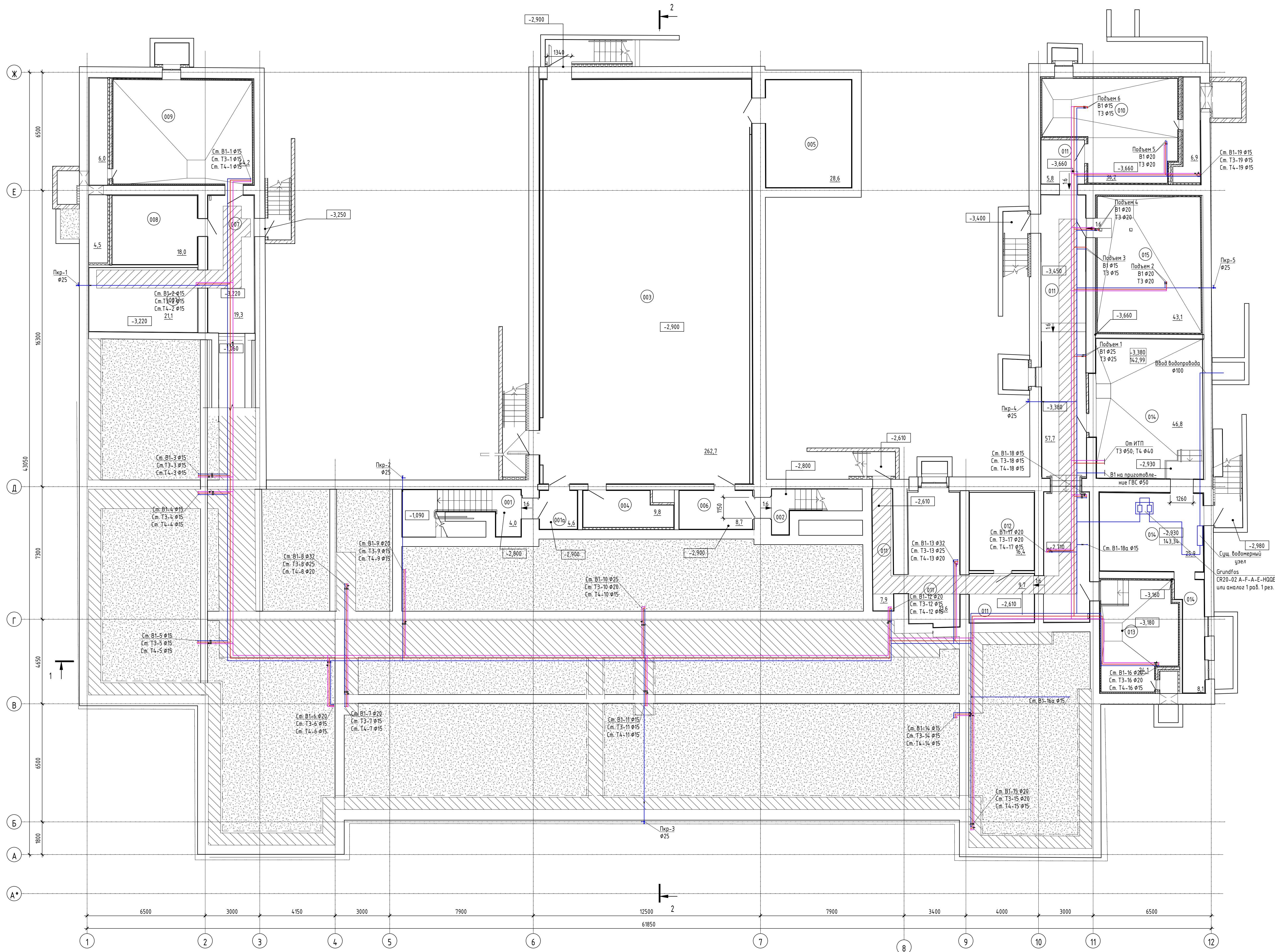
План подвала Системы водоснабжения
