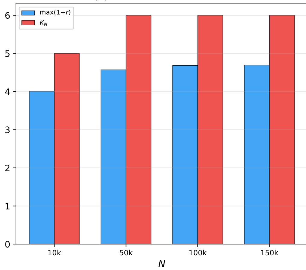
(d) Theorem 1 Verification
