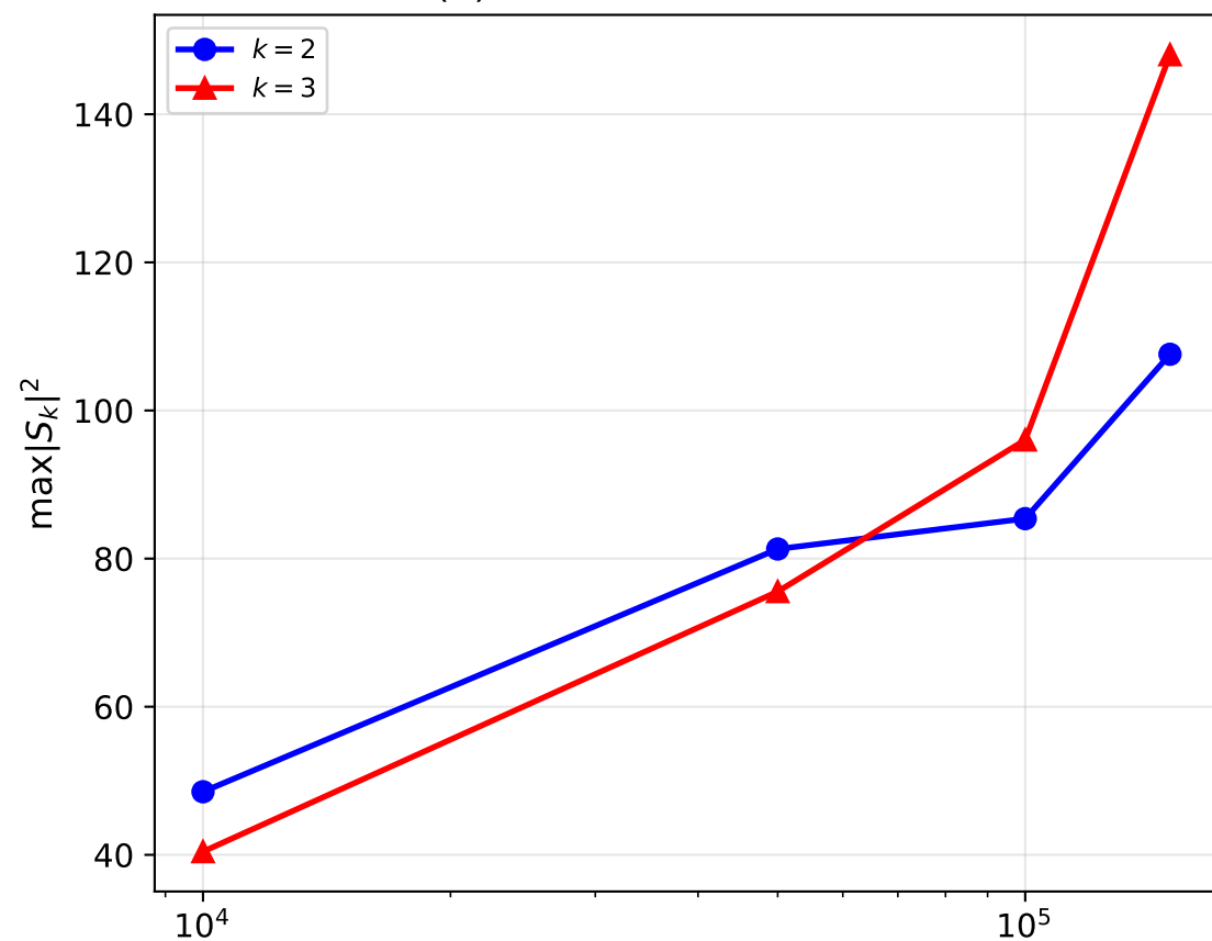
(d) Theorem 1 Verification
