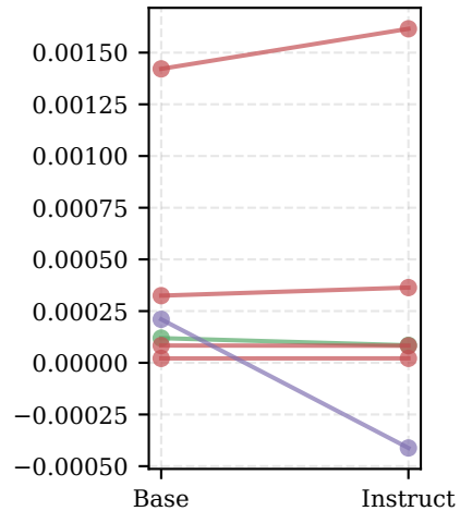
Hessian trace per param
