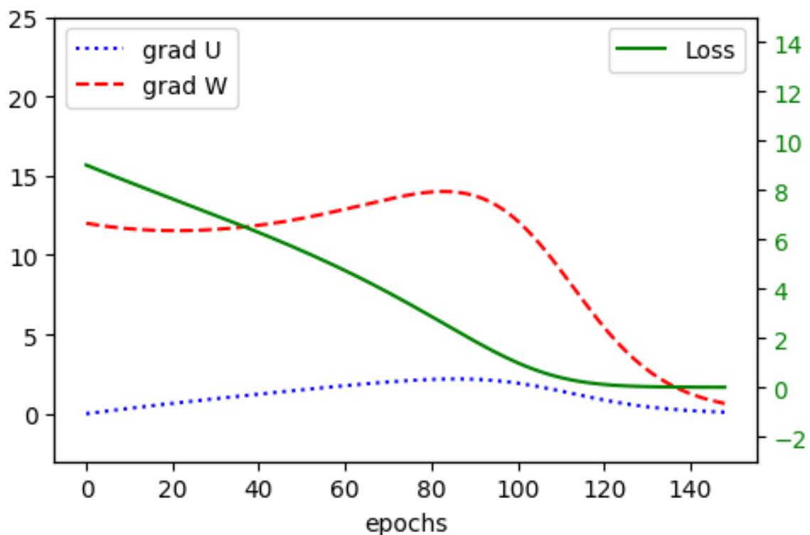
Hình 2.1: Kết quả huấn luyện với đầu vào gồm 3 số “1”.
