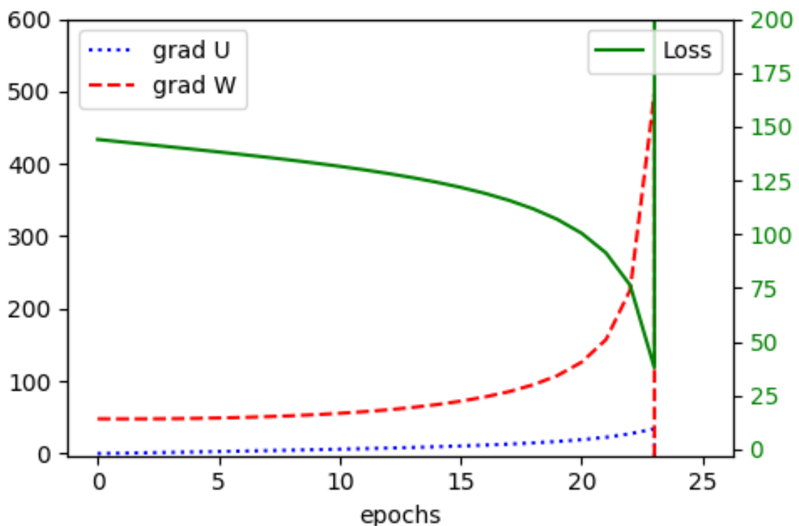
Hình 2.2: Xảy ra hiện tượng exploding trong quá trình huấn luyện.
