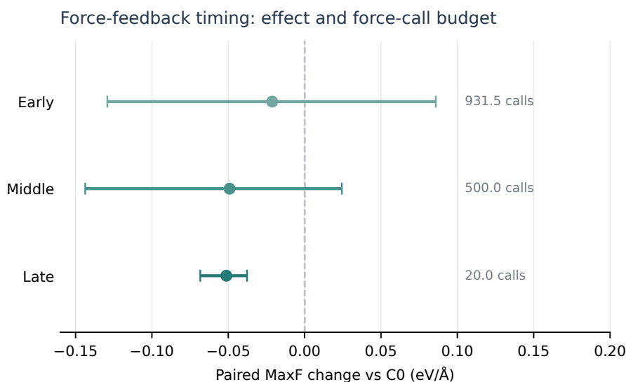
图 4-8: Timing Ablation 的配对 MatterSim MaxF 差 (候选减 C0), 点为 32 对种子的均值差, 横线为 20 000 次配对百分位自助法 95% 区间。负值表示较低代理力; Early 和 Middle 区间跨零。各臂力调用预算不同, 不构成等预算时机最优证据。
