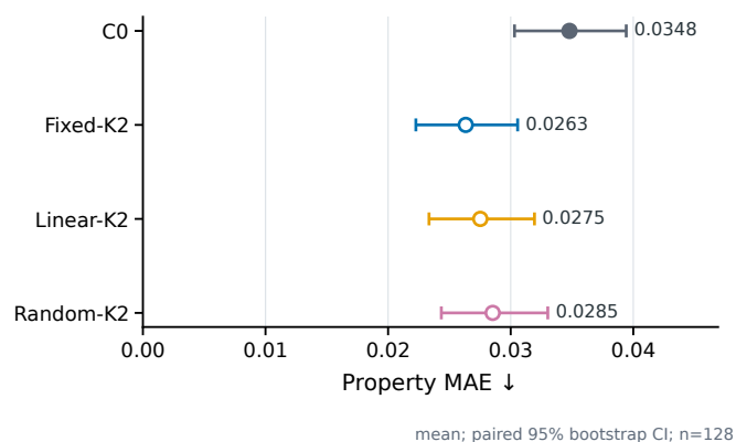
图 5-1: C1-128 四种方法的 Property MAE
