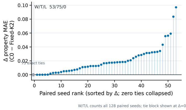
图 3-4: Fixed-K2 与 C0 的逐样本属性误差
