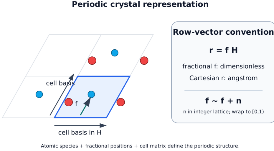
图 2-1: 晶体结构的晶胞、分数坐标与周期映射示意图
