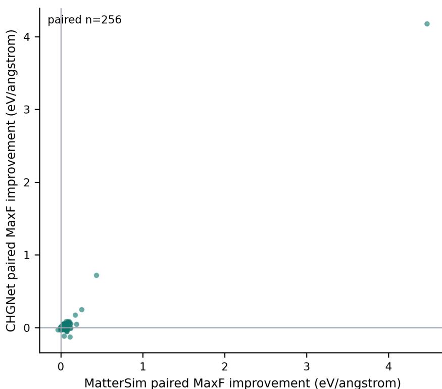
图 4-6: MatterSim 与 CHGNet 的逐样本改善比较 (release ID: I2-F5)
