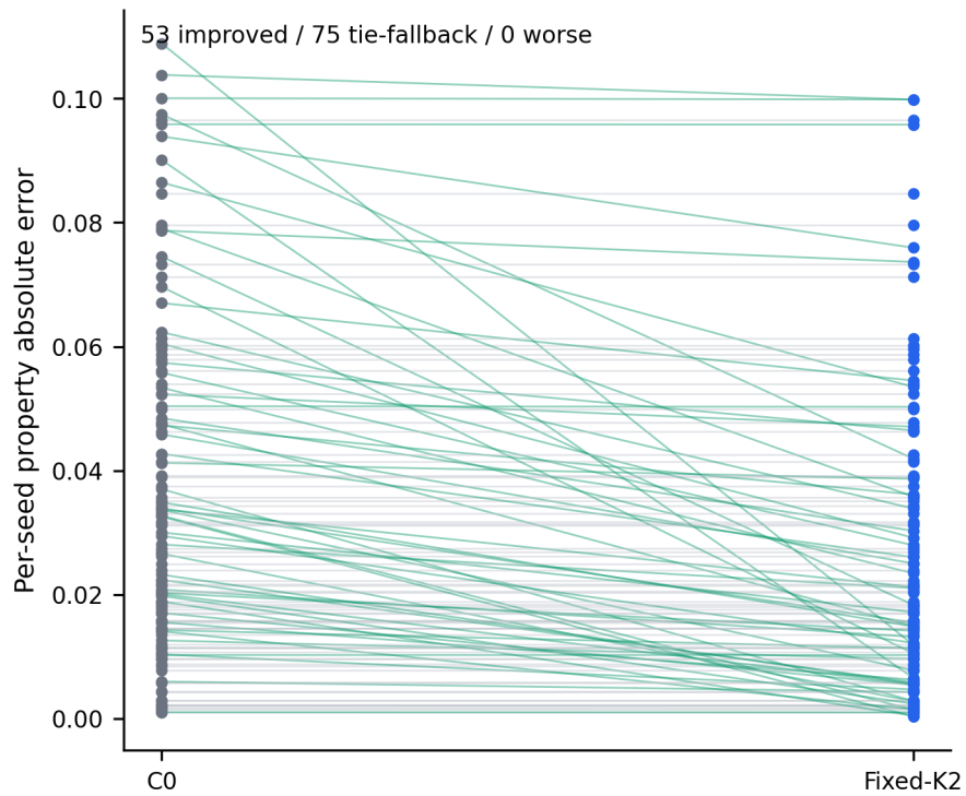
图 3-3: Fixed-K2 与 C0 的逐样本属性误差
