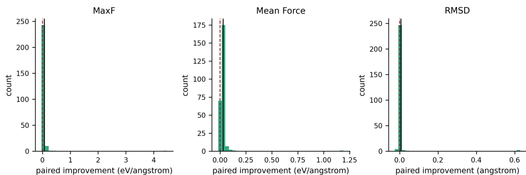
图 5-3: Formal256 配对改善分布 (release ID: I2-F3)
