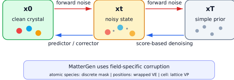
图 2-2: 扩散模型前向加噪与反向生成示意图
