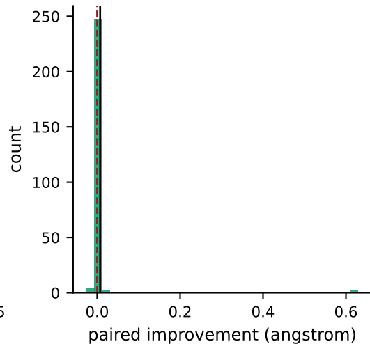
RMSD
