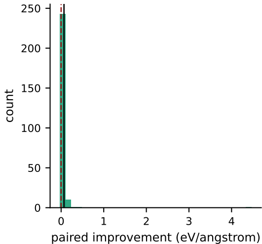
MaxF
