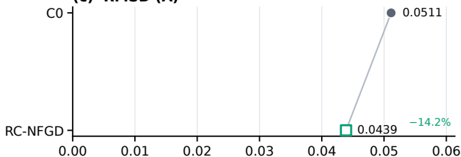
(c) RMSD (Å)
